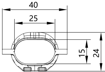
(1)标准款 允许最多安装管线：4根φ4~φ6
