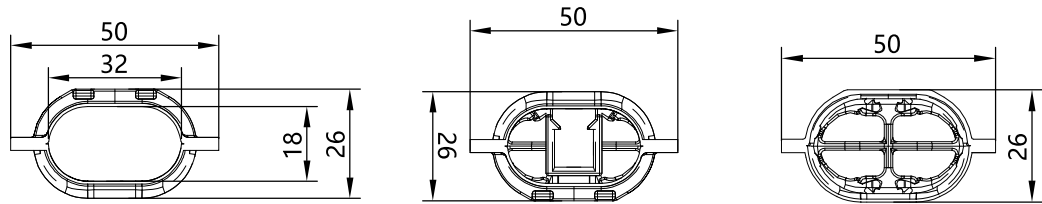
标准款 允许最多安装管线：6根*φ4 ~φ6
