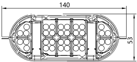
(2)带一体式分线器允许最多安装管线: 2根φ10~φ12+8根φ8~φ9+6根φ6~φ7 *分线器建议12~18个/米
