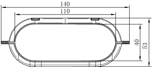
(1)标准款 允许最多安装管线: 4根φ10~φ12 +12根φ8~φ9+12根φ6~φ7
