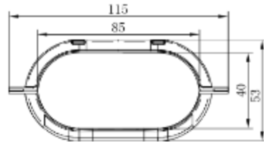
(1)标准款 允许最多安装管线: 4根φ10~φ12 + 10根φ8~φ9 + 8根φ6~φ7
