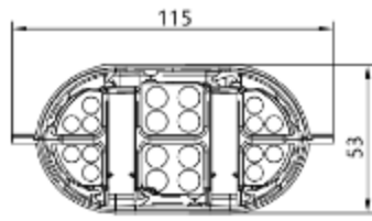
(2)带一体式分线器允许最多安装管线: 4根φ10~φ12 + 6根φ8~φ9 + 6根φ6~φ7 *分线器建议12~18个/米
