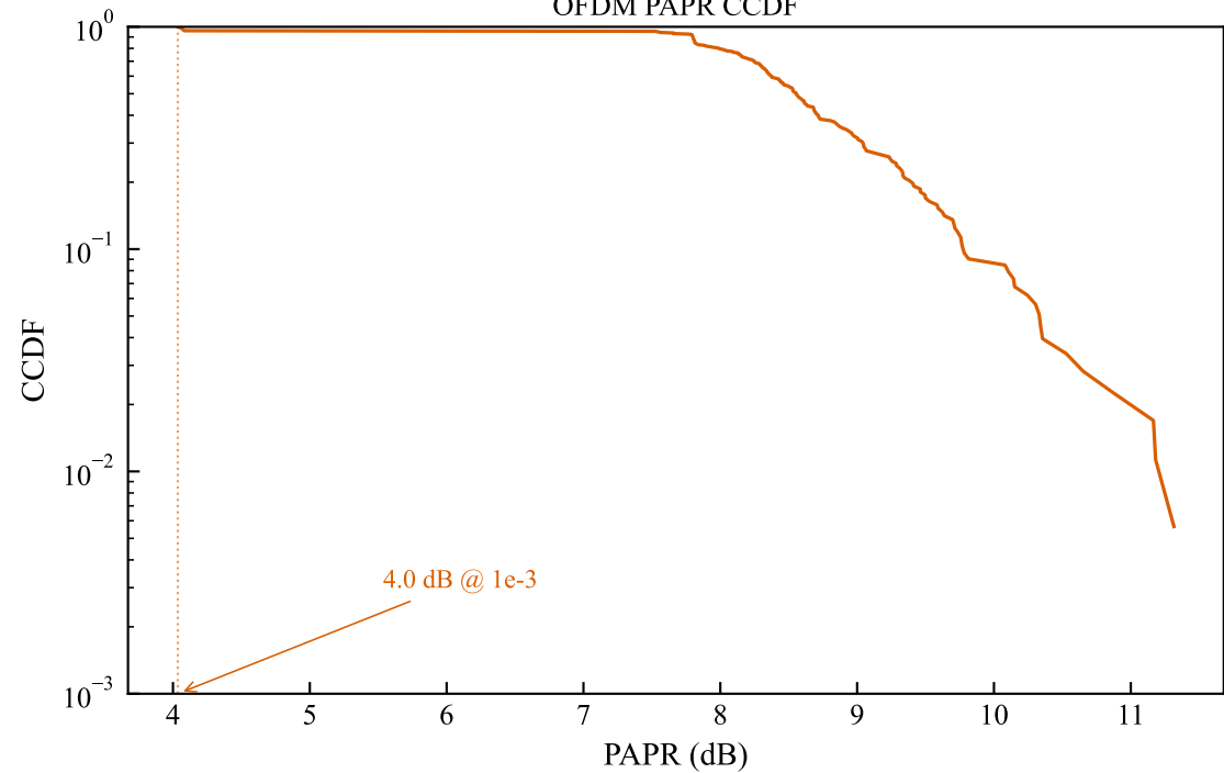
OFDM PAPR CCDF
