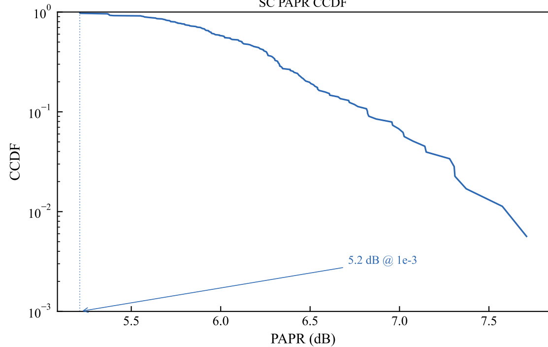
SC PAPR CCDF
