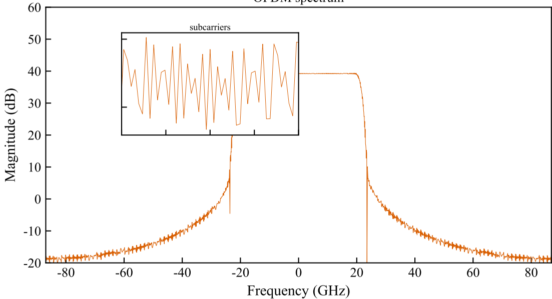
OFDM spectrum
