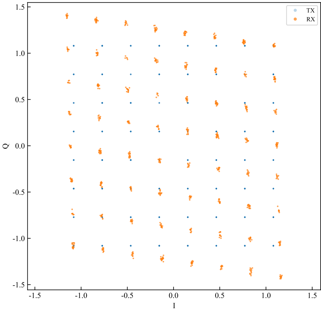
SC-FDE — iq_no_comp
