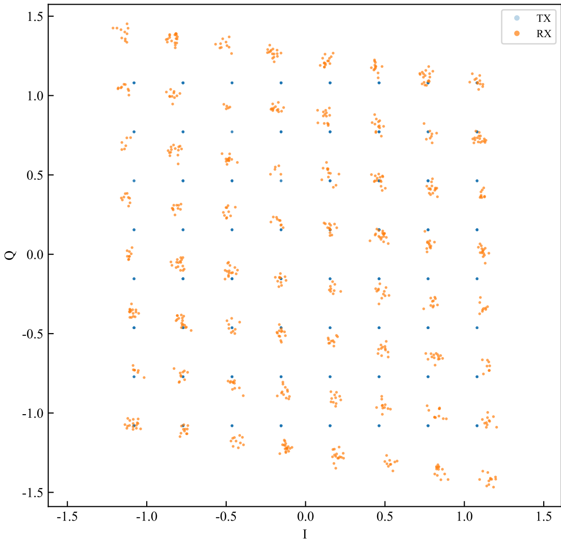
SC-FDE — iq_no_comp
