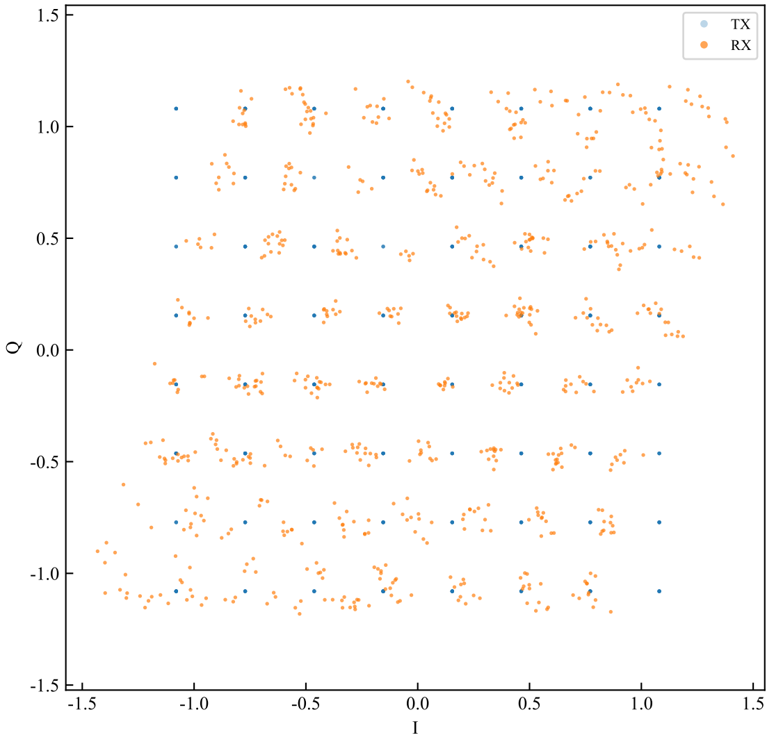
SC-FDE — iq_comp
