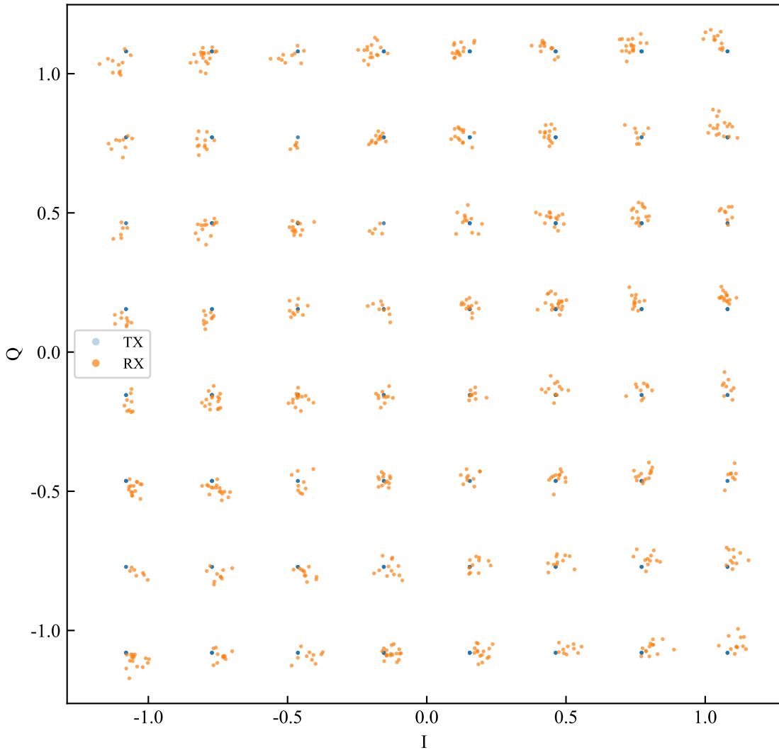
SC-FDE — no_iq
