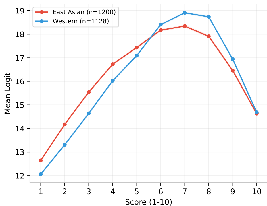
Llama
