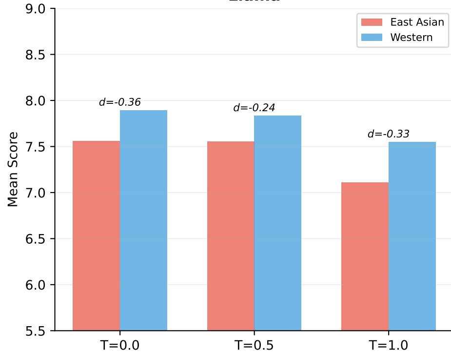
Llama
