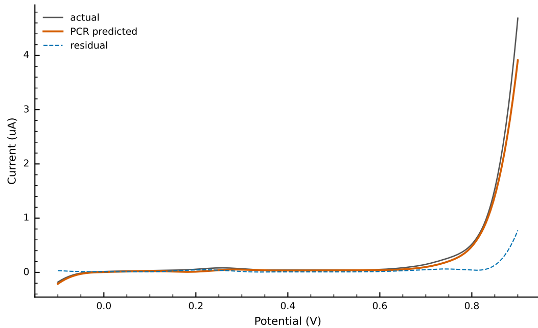
CV GC - Anodic
