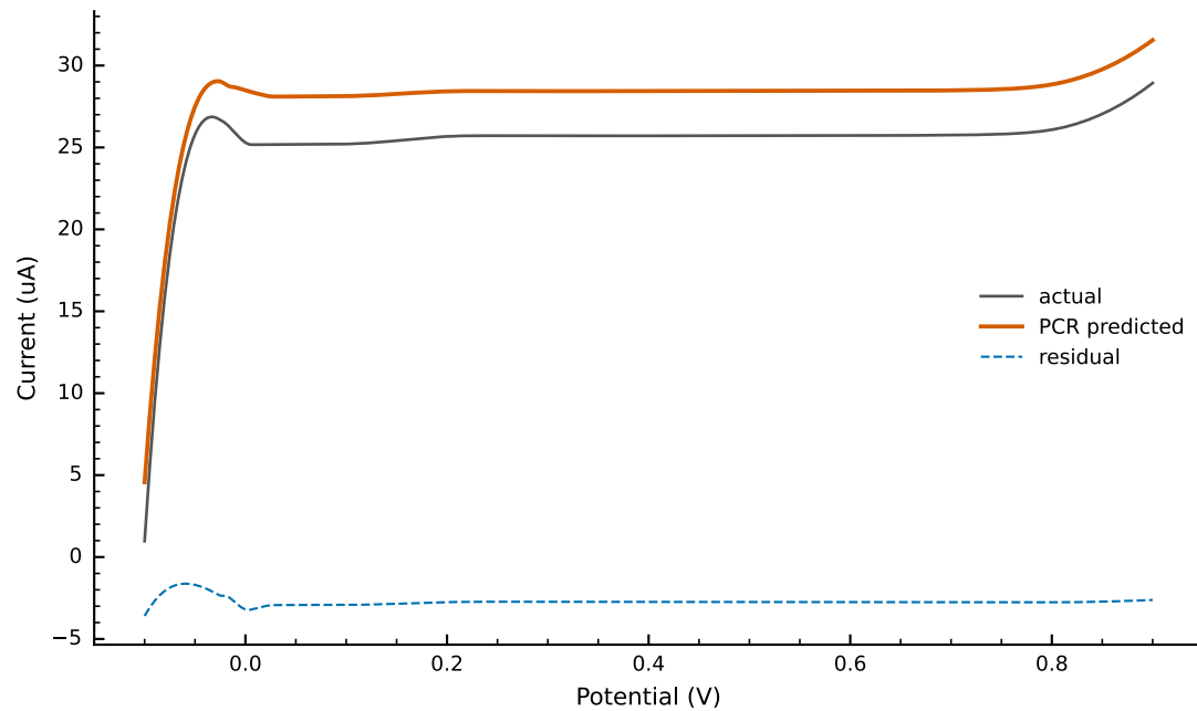
CV GC - Anodic
