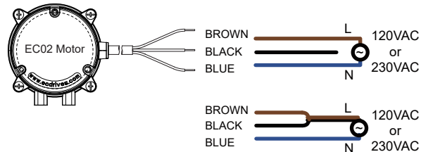
ECY-02 Wiring Schematic
