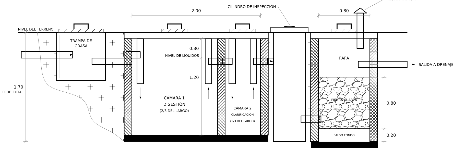
ESQUEMA: LA TRAMPA DE GRASA SE UBICA EN EL COLECTOR AG Y LAS AGUAS NEGRAS ENTRAN POR LA CR DE ENTRADA (VER PLANTA N1).
