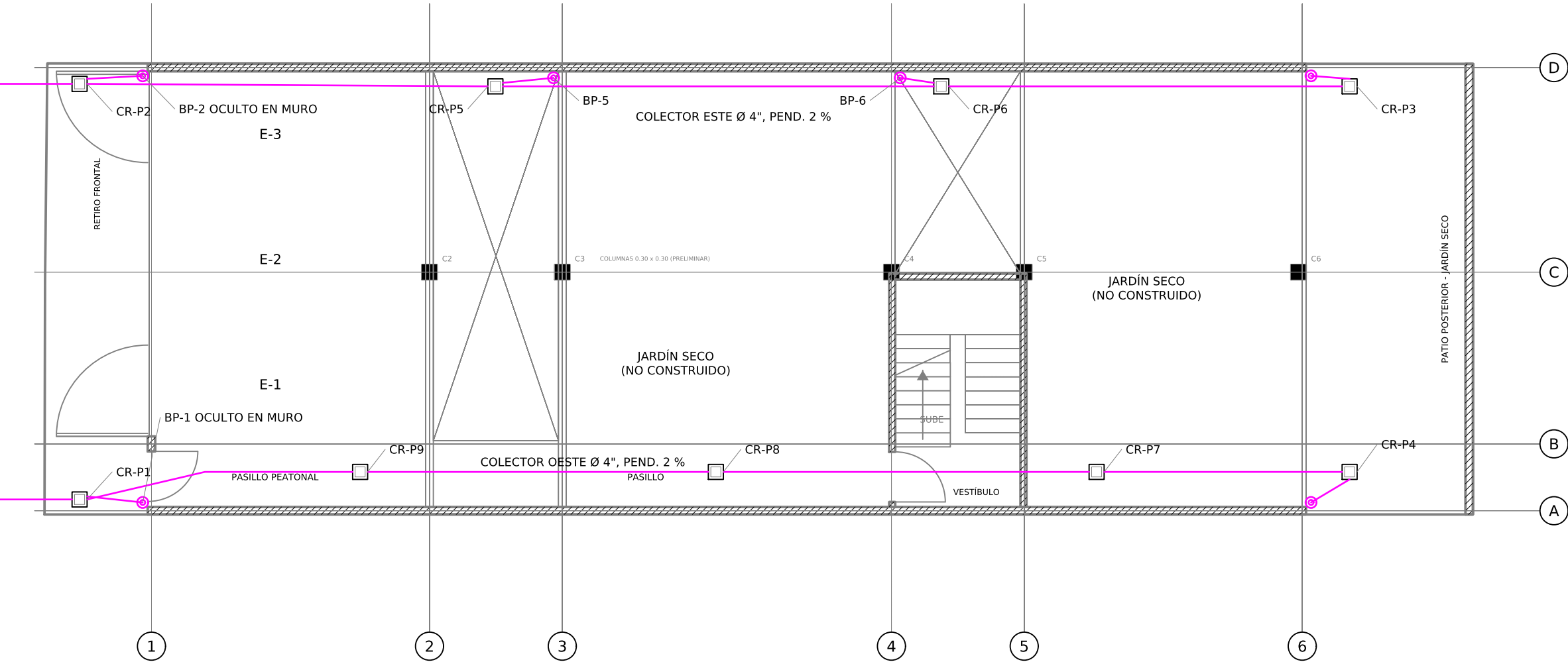
AGUAS PLUVIALES - NIVEL 1 Esc. 1:100
