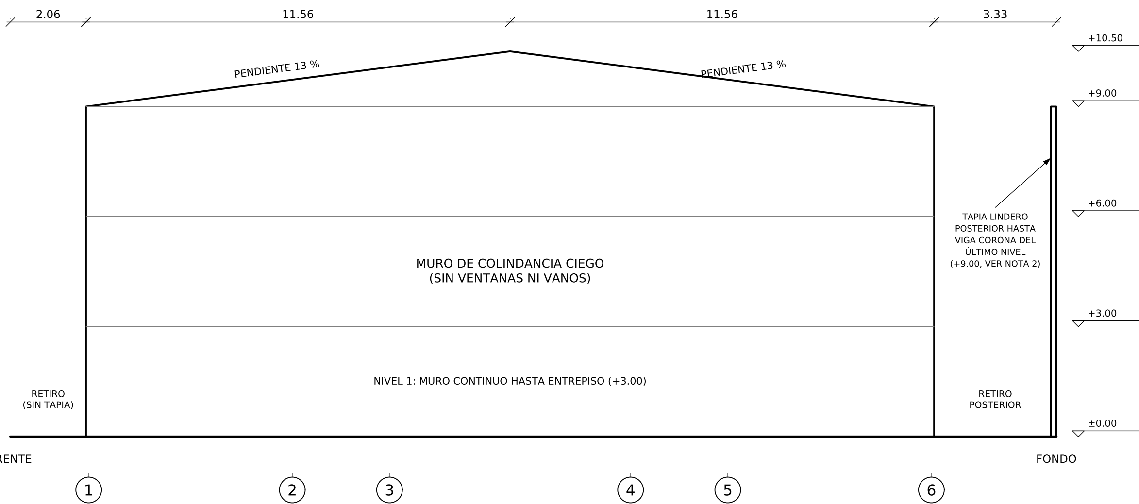
FACHADA LATERAL OESTE MURO DE COLINDANCIA Esc. 1:100
