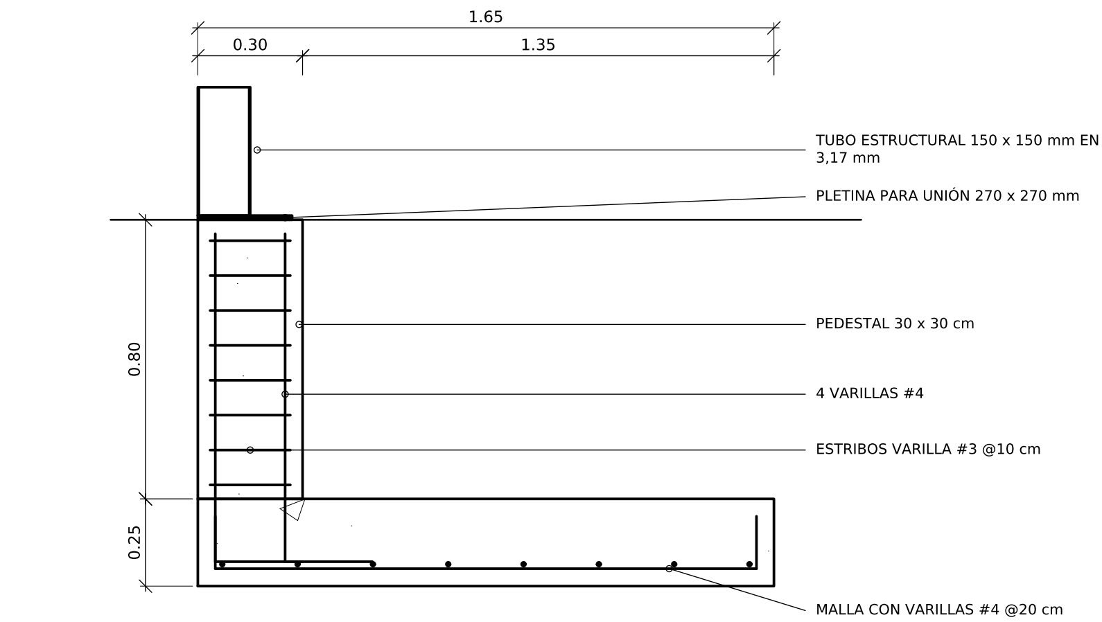
CORTE FUNDACIÓN F2 (EXCÉNTRICA, LINDERO) Esc. 1:15
