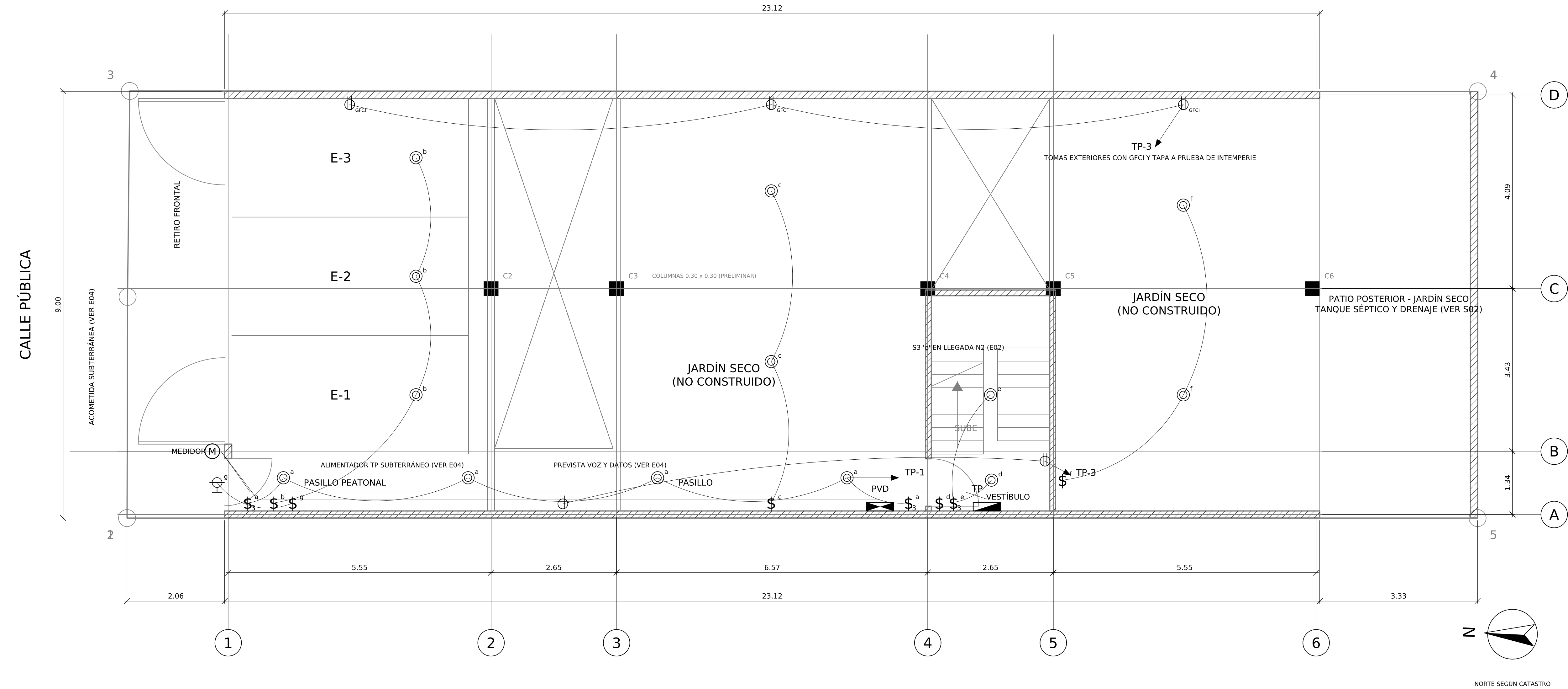
PLANTA ELÉCTRICA NIVEL 1 ILUMINACIÓN, TOMACORRIENTES Y VOZ/DATOS Esc. 1:50
