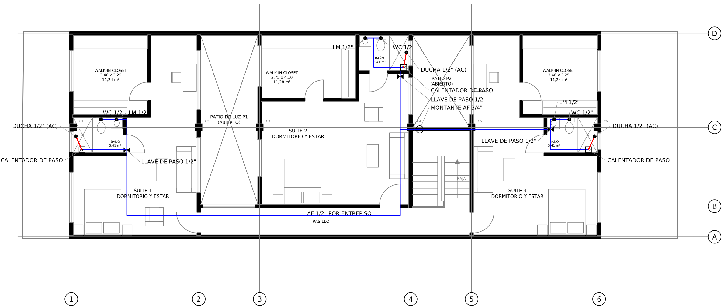
AGUA POTABLE - NIVEL 3 Esc. 1:100
