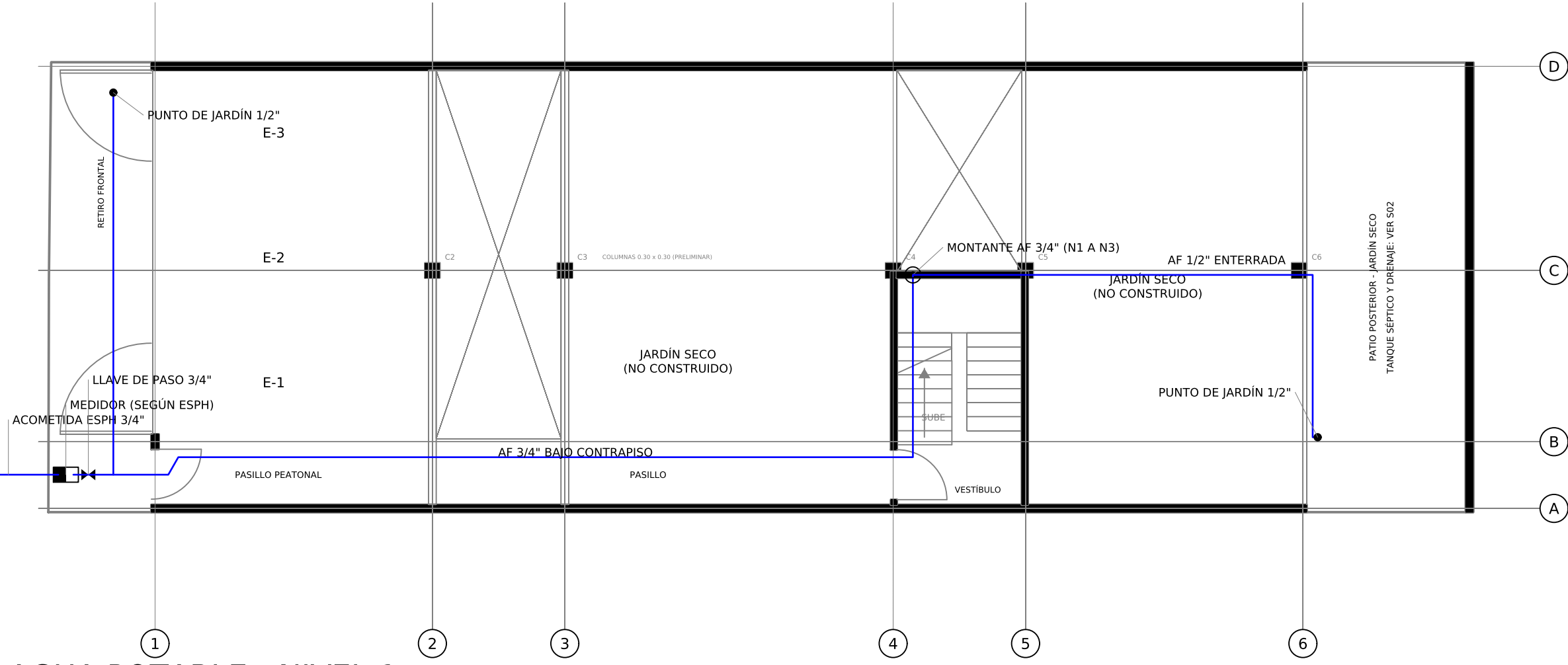
AGUA POTABLE - NIVEL 1 Esc. 1:100
