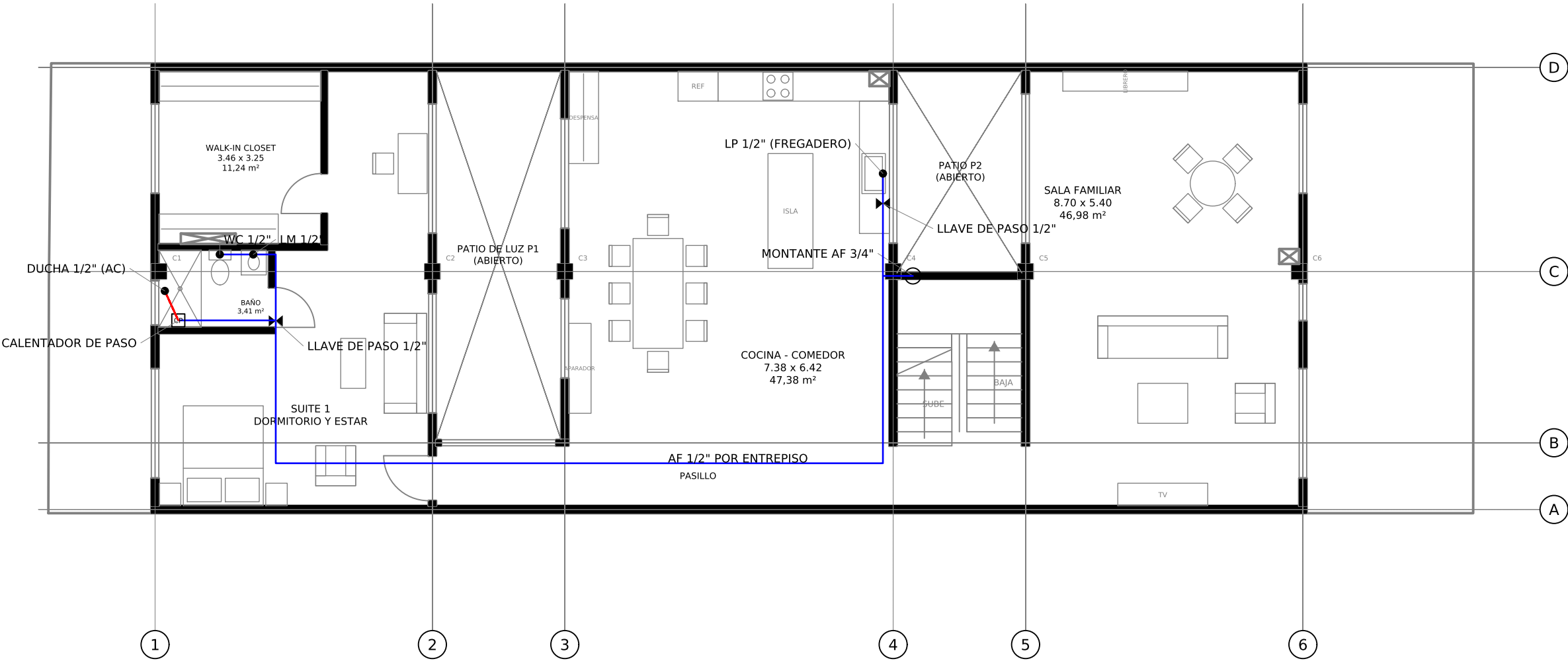
AGUA POTABLE - NIVEL 2 Esc. 1:100
