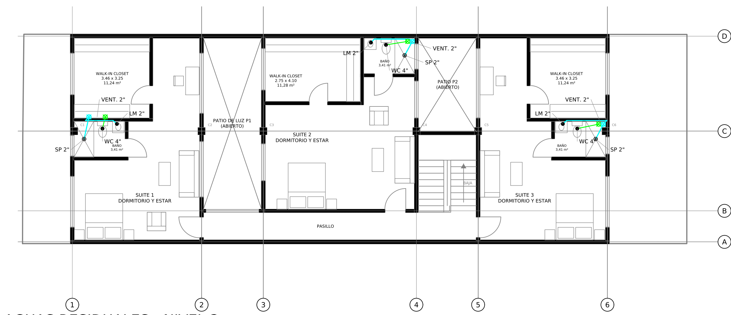
AGUAS RESIDUALES - NIVEL 3 Esc. 1:100
