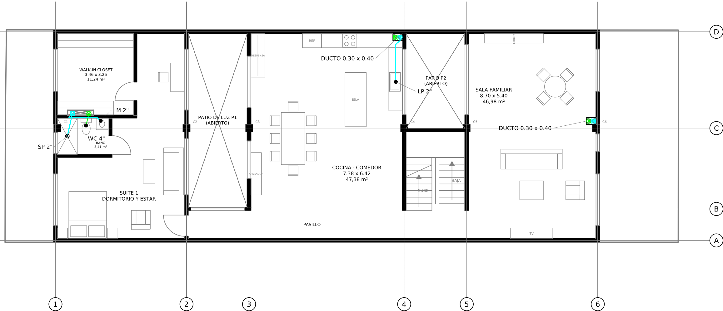
AGUAS RESIDUALES - NIVEL 2 Esc. 1:100
