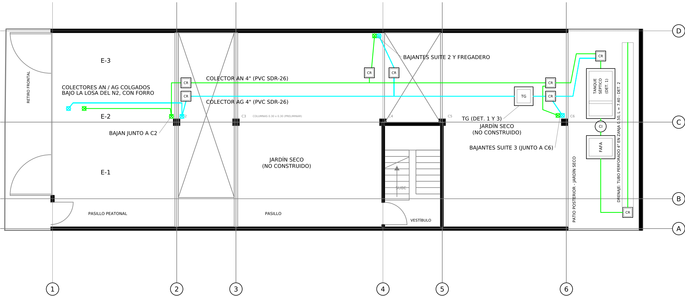
AGUAS RESIDUALES - NIVEL 1 Esc. 1:100
