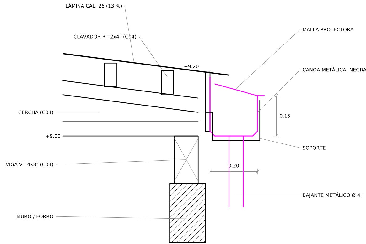
DETALLE 1 - CANOA (SECCIÓN TÍPICA) Esc. 1:10 - FRONTAL, POSTERIOR Y HACIA PATIOS
