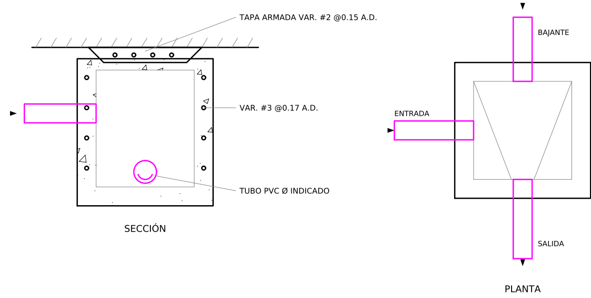
DETALLE 3 - DESCARGA A CUNETA (ESQUEMÁTICO) S/E
