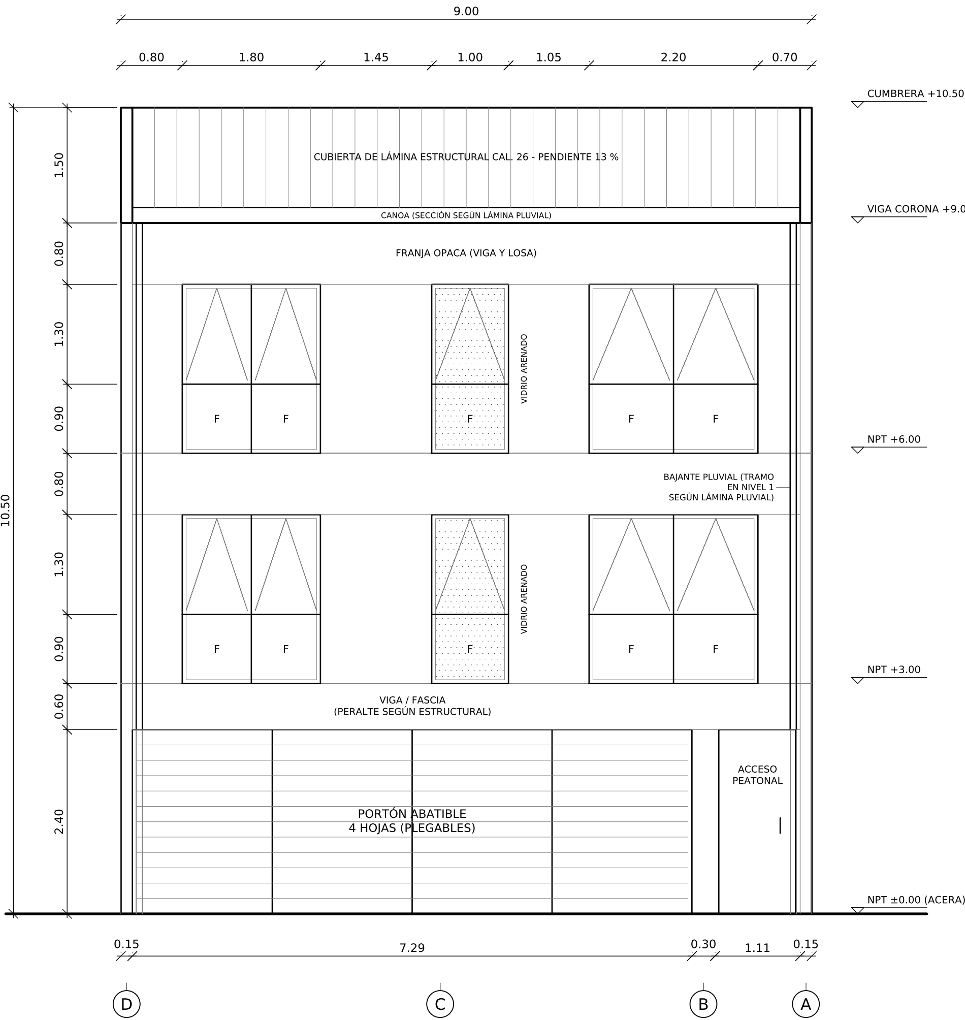
FACHADA PRINCIPAL (NORTE) VISTA DESDE LA CALLE Esc. 1:50
