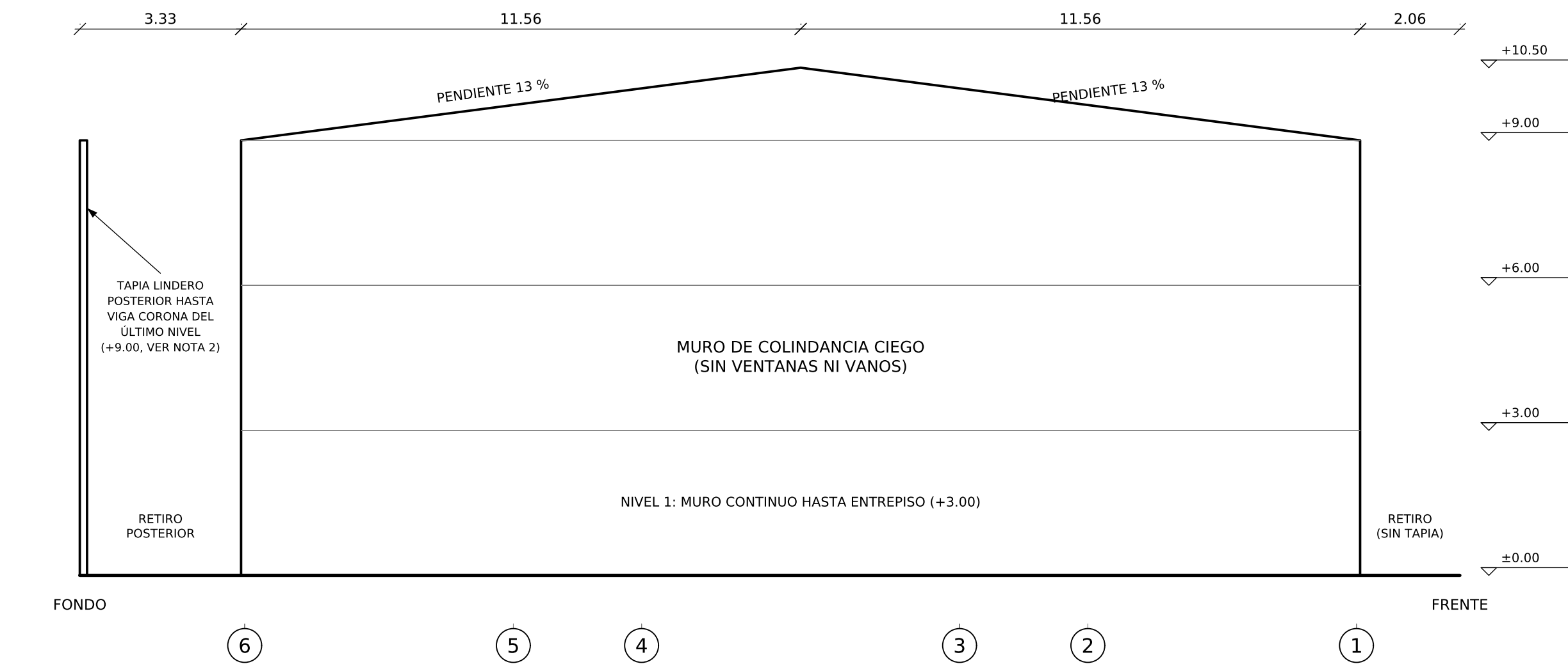
FACHADA LATERAL ESTE MURO DE COLINDANCIA Esc. 1:100
