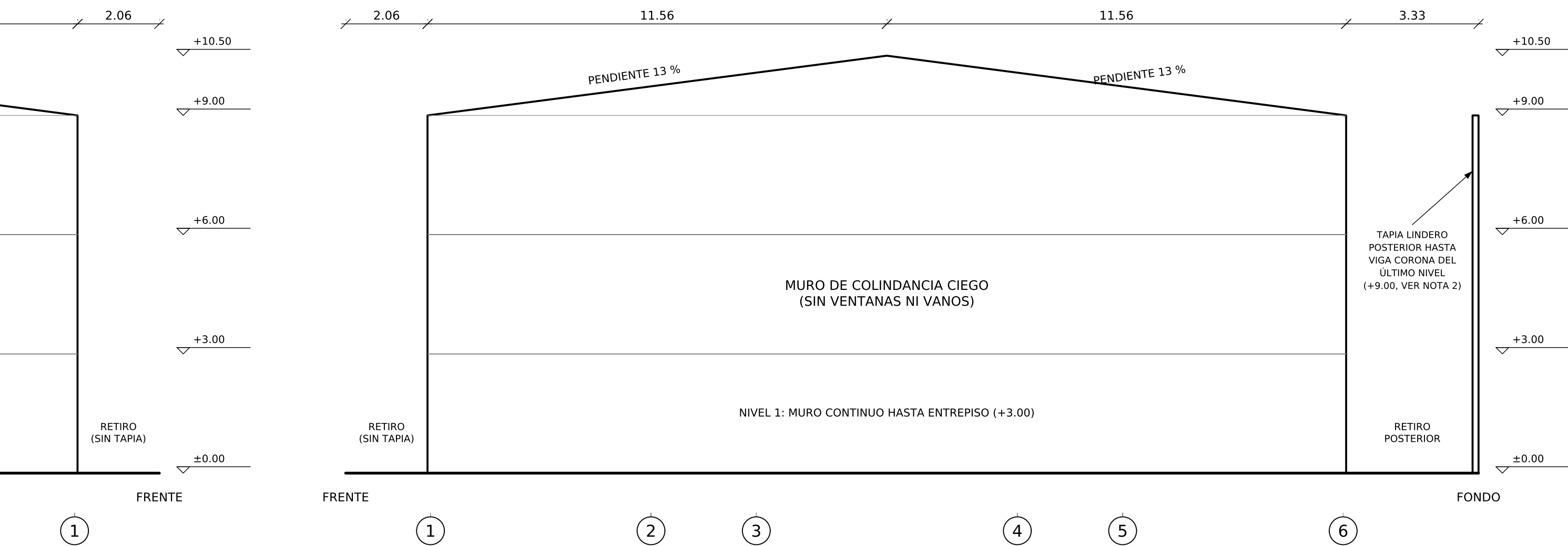
FACHADA LATERAL OESTE MURO DE COLINDANCIA Esc. 1:100
