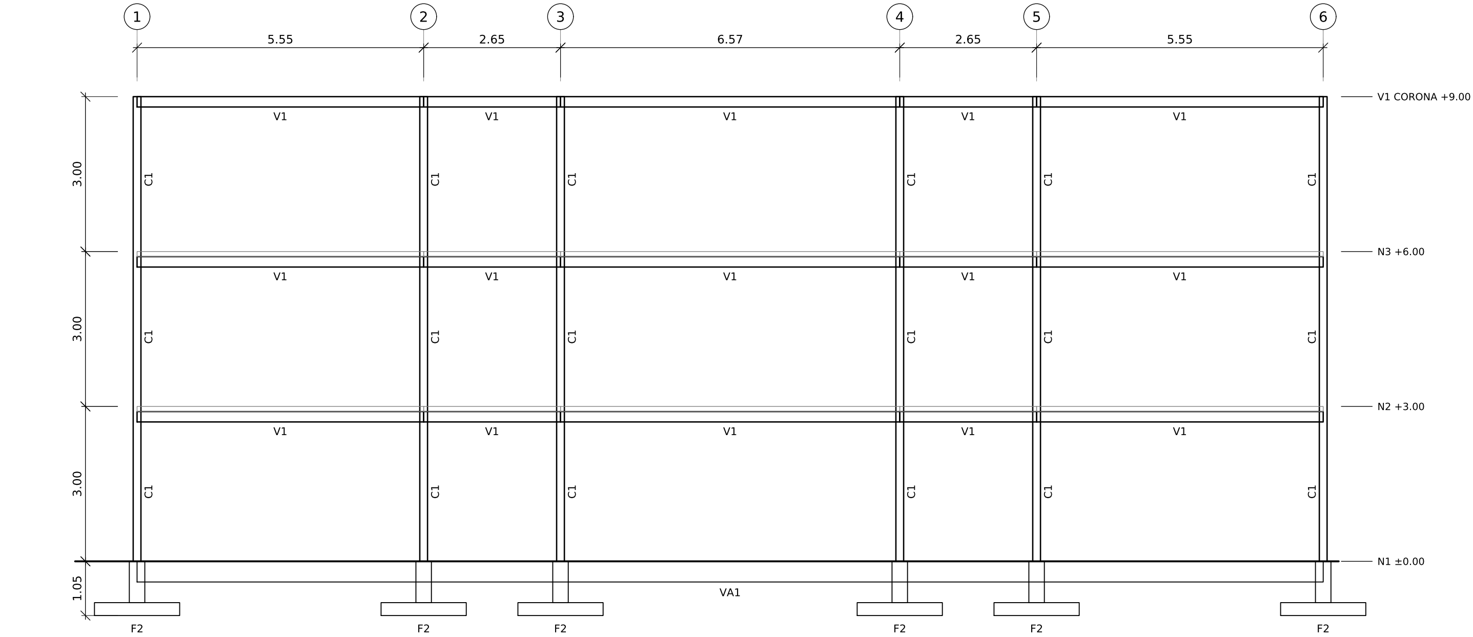
PÓRTICOS A Y D EJES 1 A 6 (COLINDANCIAS) - Esc. 1:75
