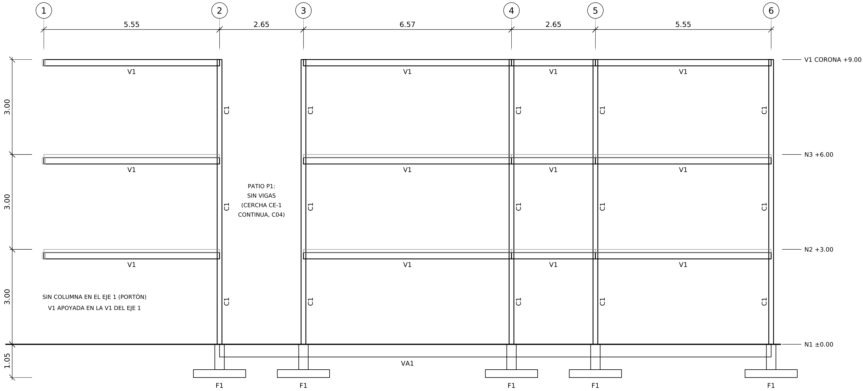
PÓRTICO C EJES 1 A 6 (COLUMNAS FORRADAS A 0,30 x 0,30) - Esc. 1:75
