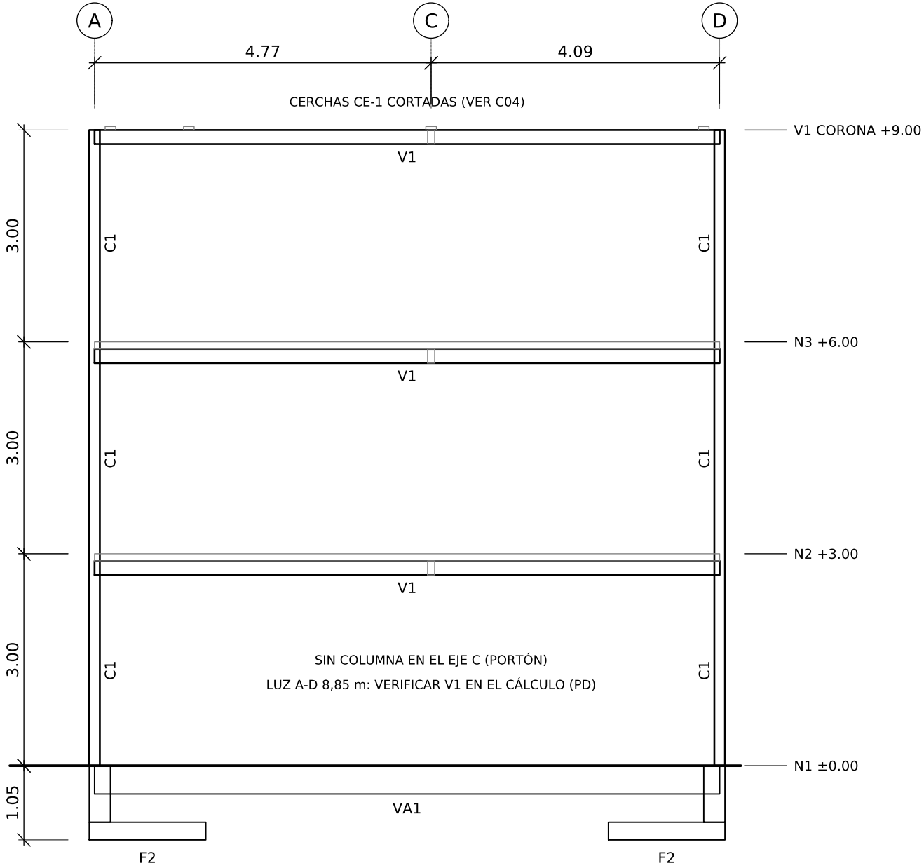
PÓRTICO 1
