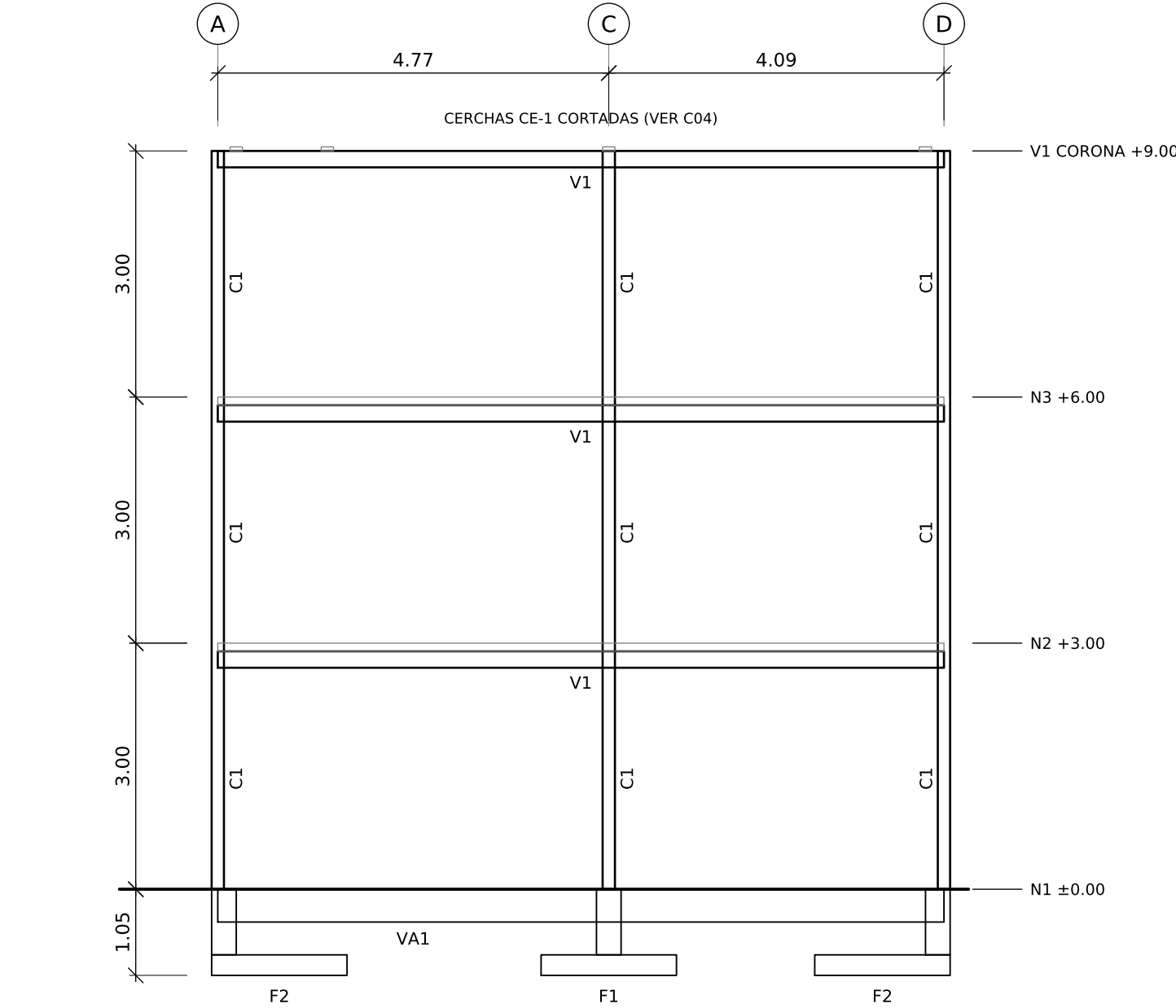
PÓRTICOS 2 A 6
