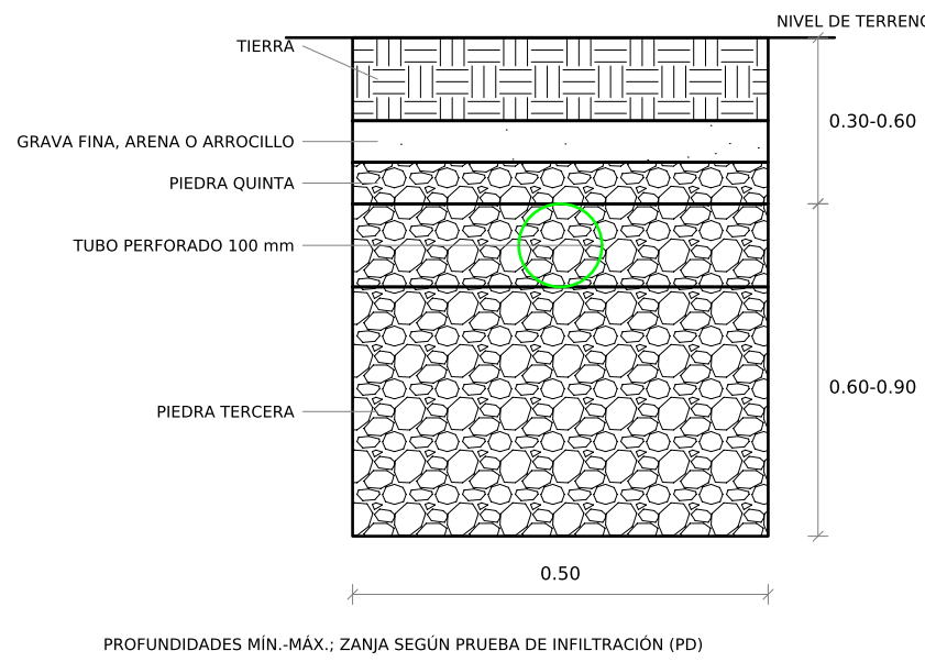
PROFUNDIDADES MIN.-MAX.; ZANJA SEGÚN PRUEBA DE INFILTRACIÓN (PD)
