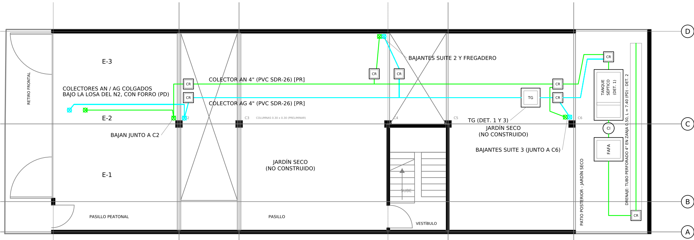
AGUAS RESIDUALES - NIVEL 2 Esc. 1:100
