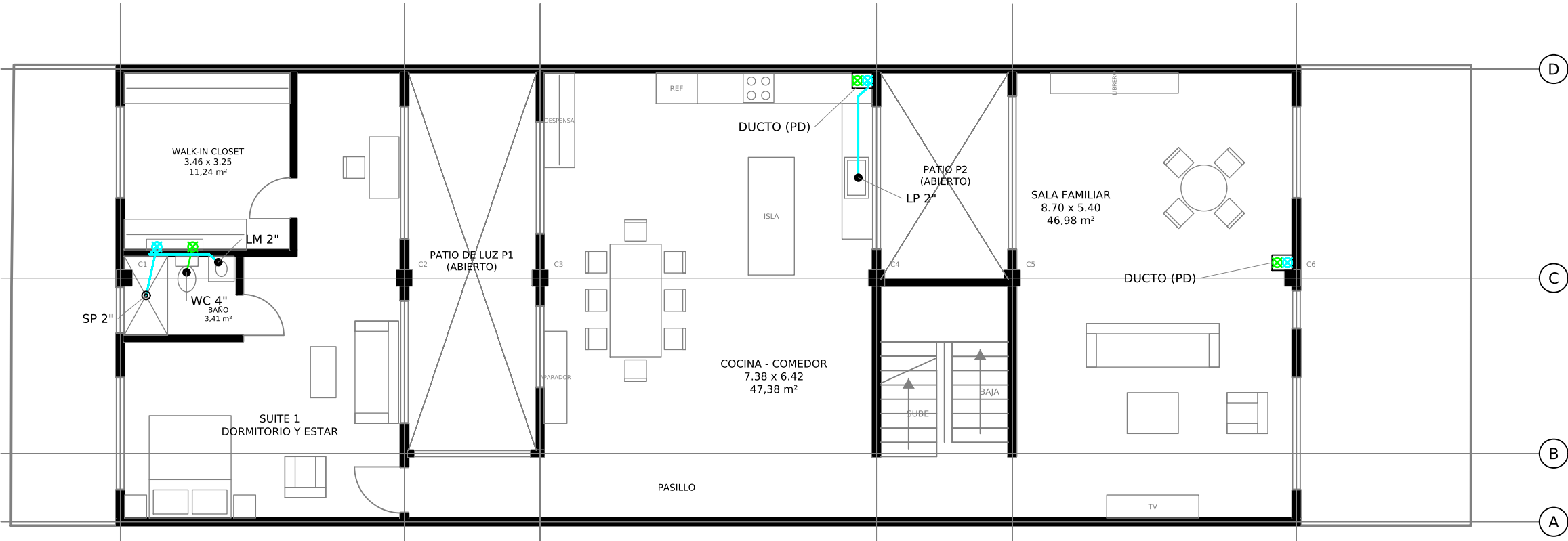
AGUAS RESIDUALES - NIVEL 3 Esc. 1:100
