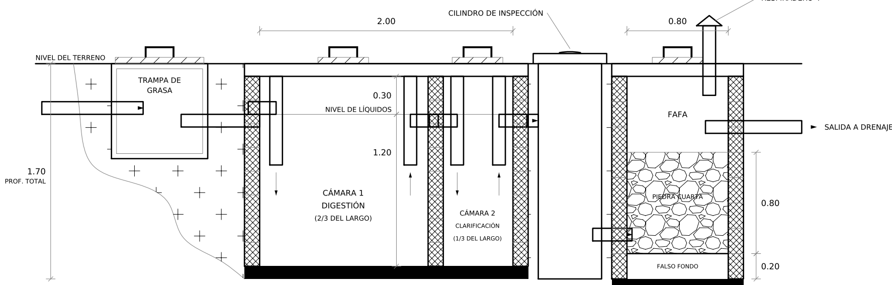
ESQUEMA: LA TRAMPA DE GRASA SE UBICA EN EL COLECTOR AG Y LAS AGUAS NEGRAS ENTRAN POR LA CR DE ENTRADA (VER PLANTA N1).
