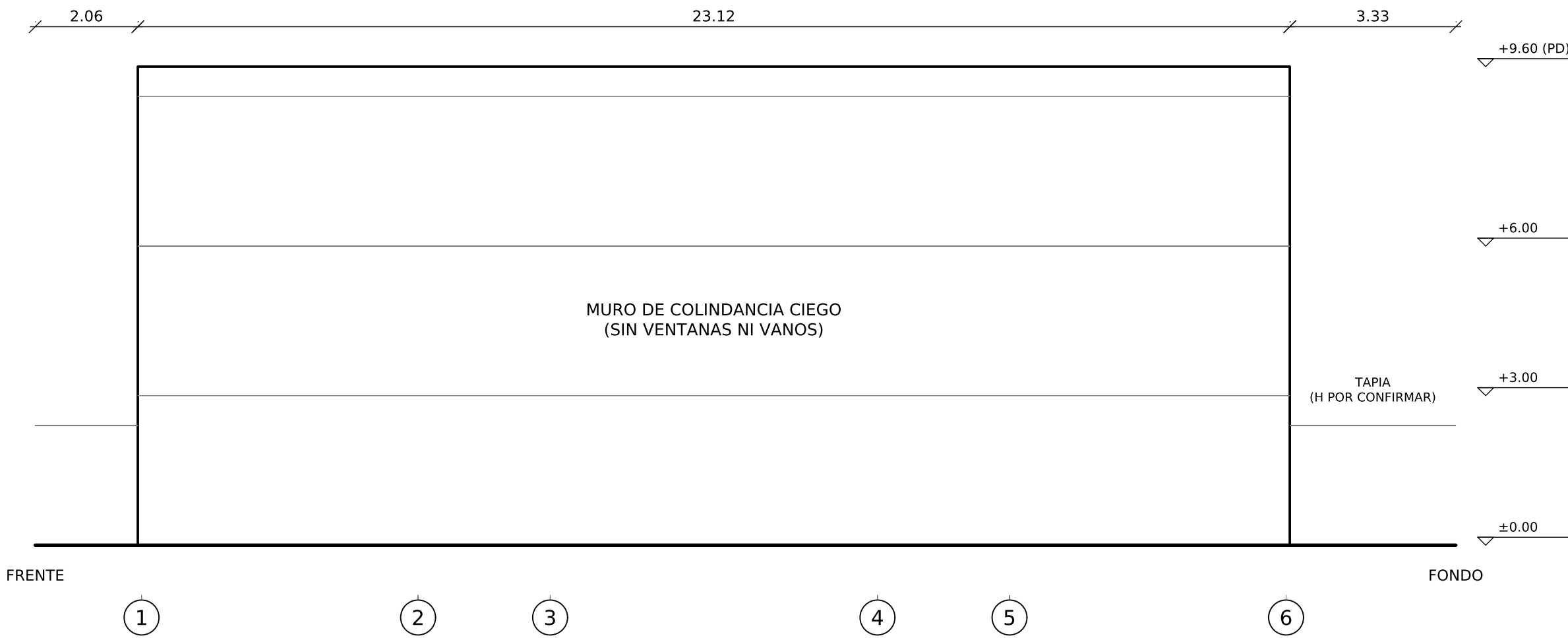
FACHADA LATERAL OESTE MURO DE COLINDANCIA Esc. 1:100
