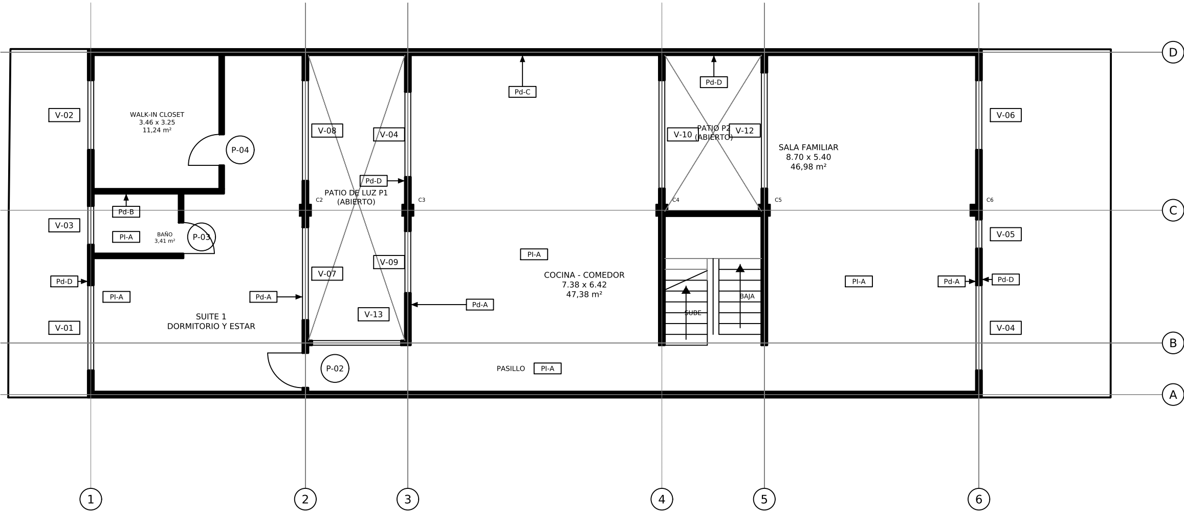
PLANTA NIVEL 2 PUERTAS, VENTANAS Y ACABADOS - Esc. 1:100
