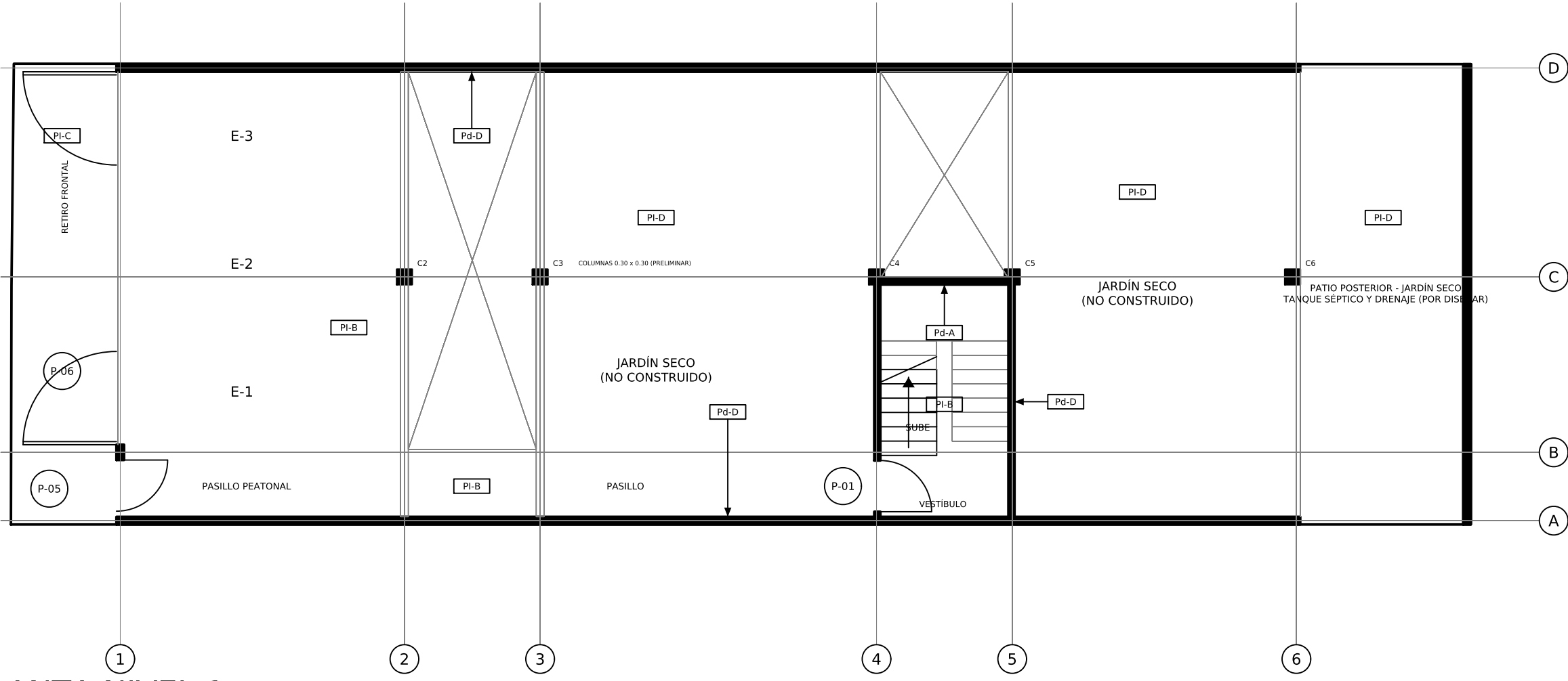
PLANTA NIVEL 1 PUERTAS, VENTANAS Y ACABADOS - Esc. 1:100
