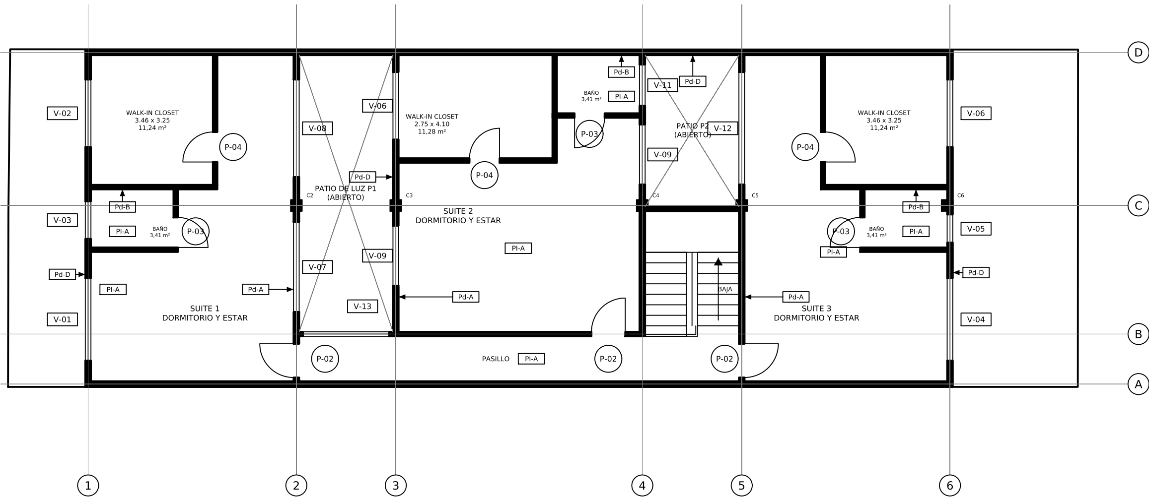
PLANTA NIVEL 3 PUERTAS, VENTANAS Y ACABADOS - Esc. 1:100
