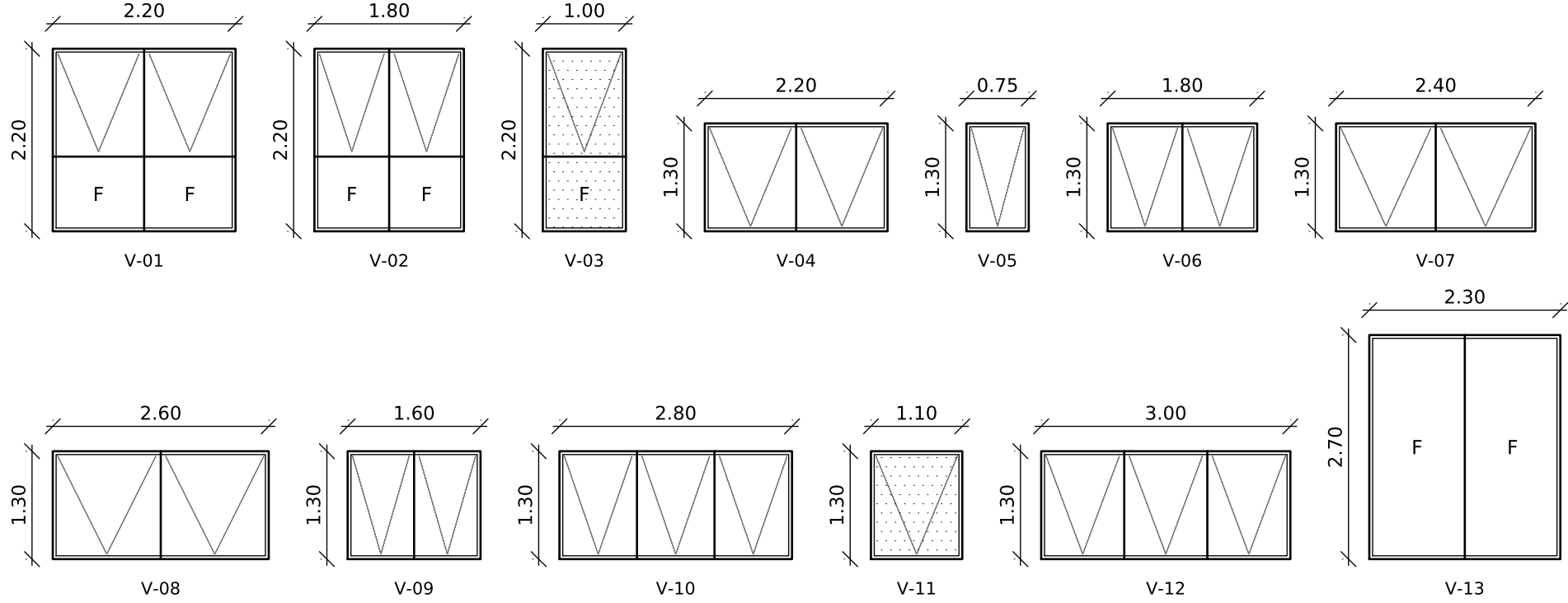
DETALLE VENTANAS Esc. 1:75 - VISTA EXTERIOR
