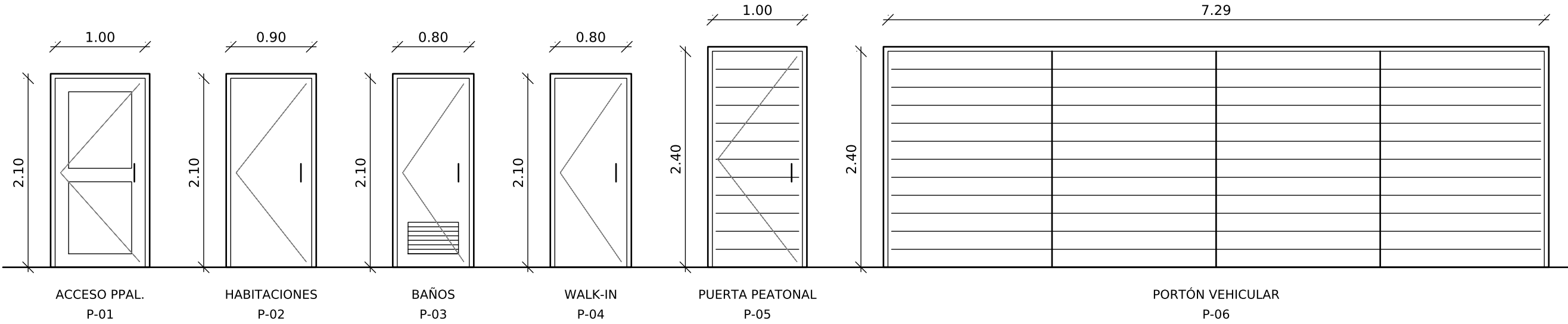
DETALLE PUERTAS Esc. 1:50 - VISTA DESDE EL LADO DE APERTURA
