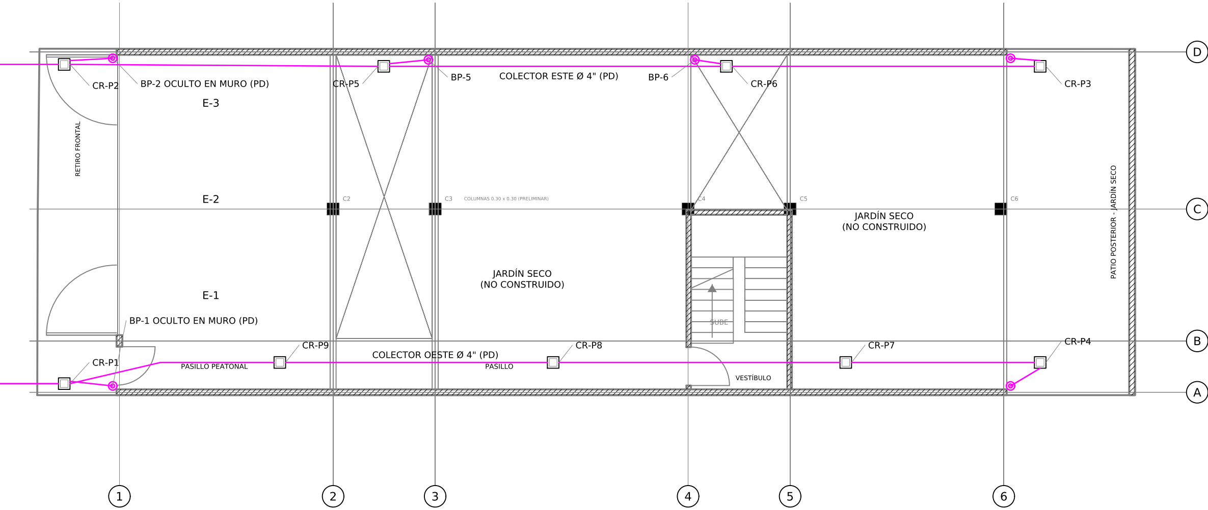
AGUAS PLUVIALES - NIVEL 1 Esc. 1:100
