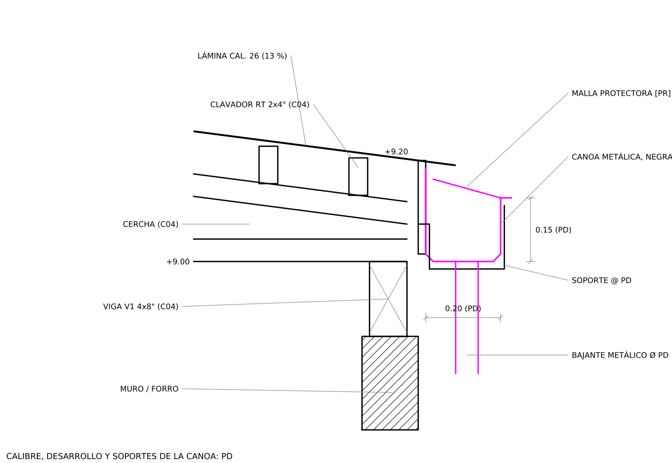
DETALLE 1 - CANOA (SECCIÓN TÍPICA) Esc. 1:10 - FRONTAL, POSTERIOR Y HACIA PATIOS
