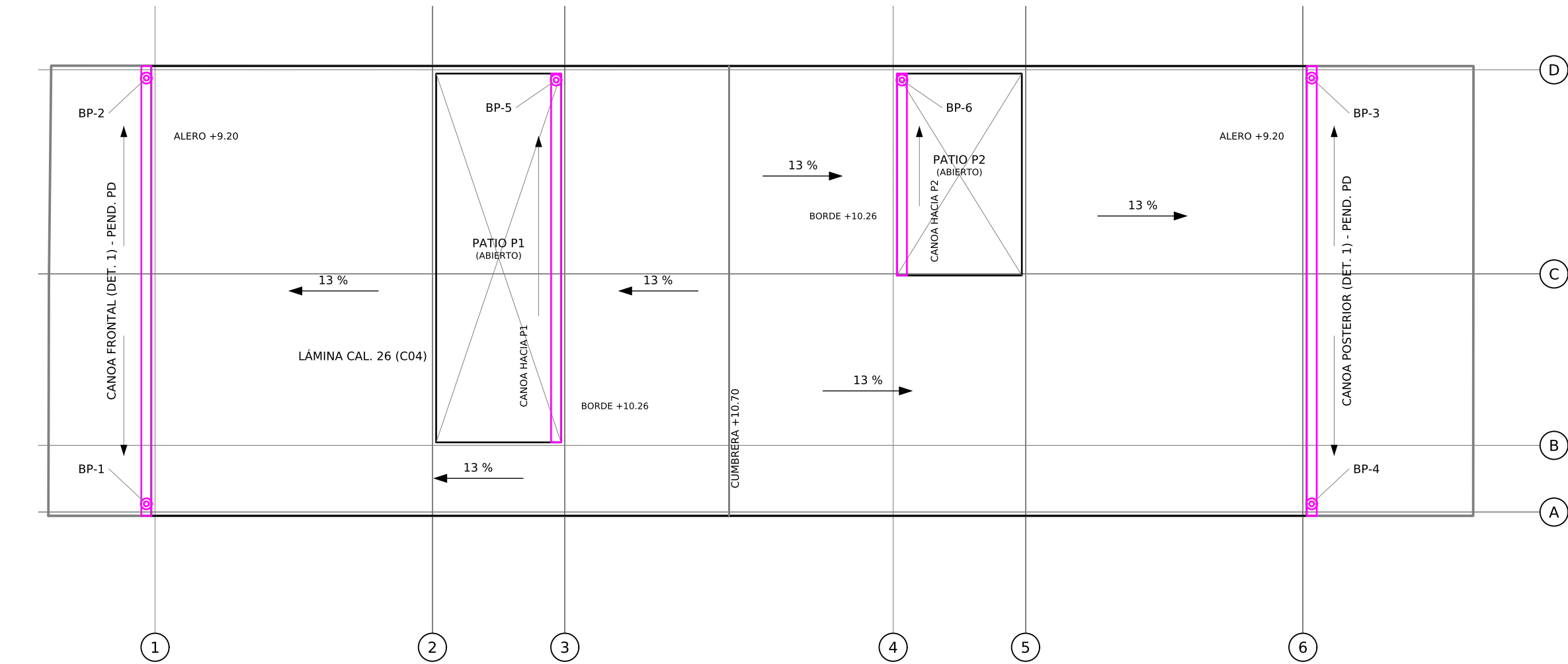
AGUAS PLUVIALES - PLANTA DE TECHO Esc. 1:100
