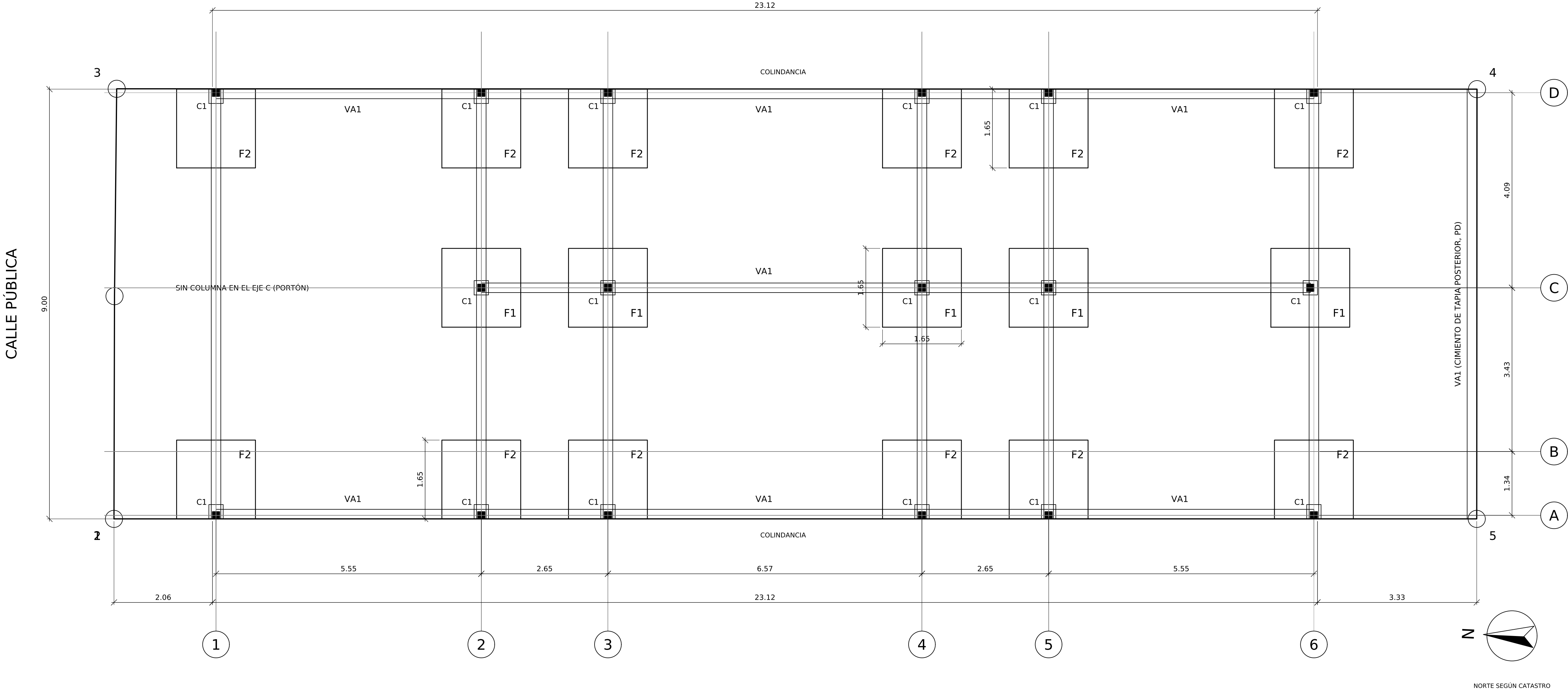
CUADRO DE CIMENTACIONES
