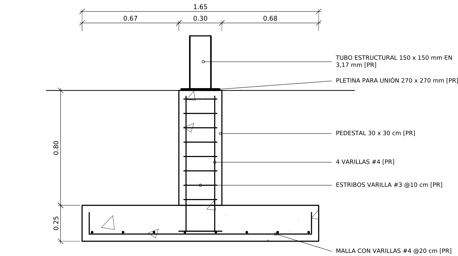
CORTE FUNDACIÓN F1 (CENTRADA) Esc. 1:15
