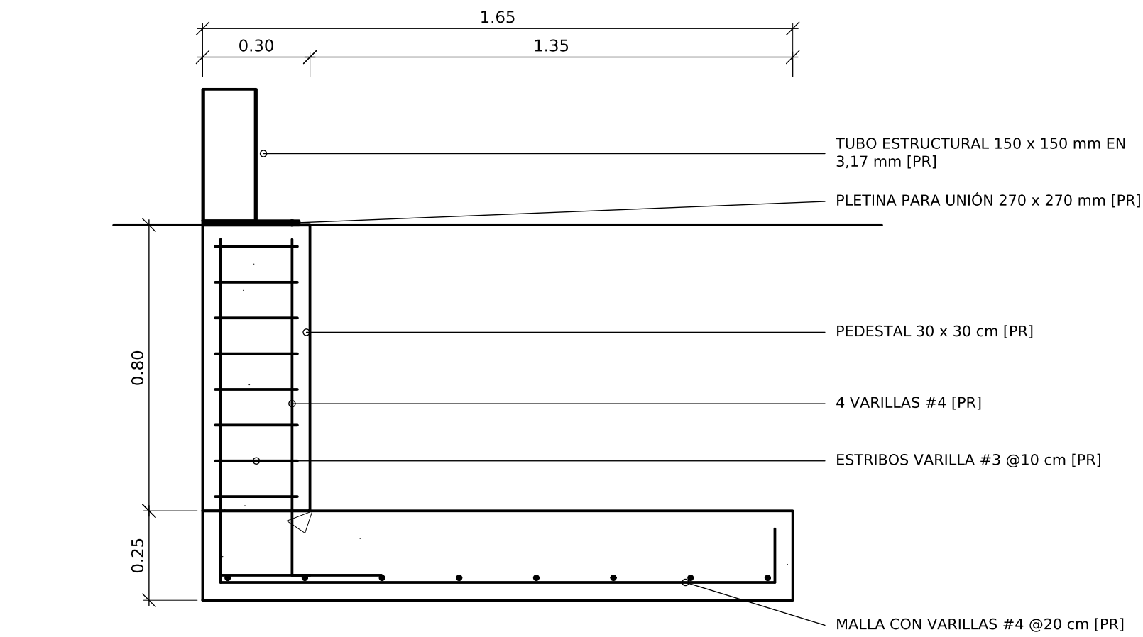
CORTE FUNDACIÓN F2 (EXCÉNTRICA, LINDERO) Esc. 1:15
