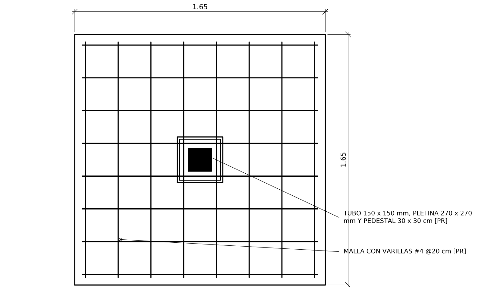
PLANTA FUNDACIÓN F1 Esc. 1:15
