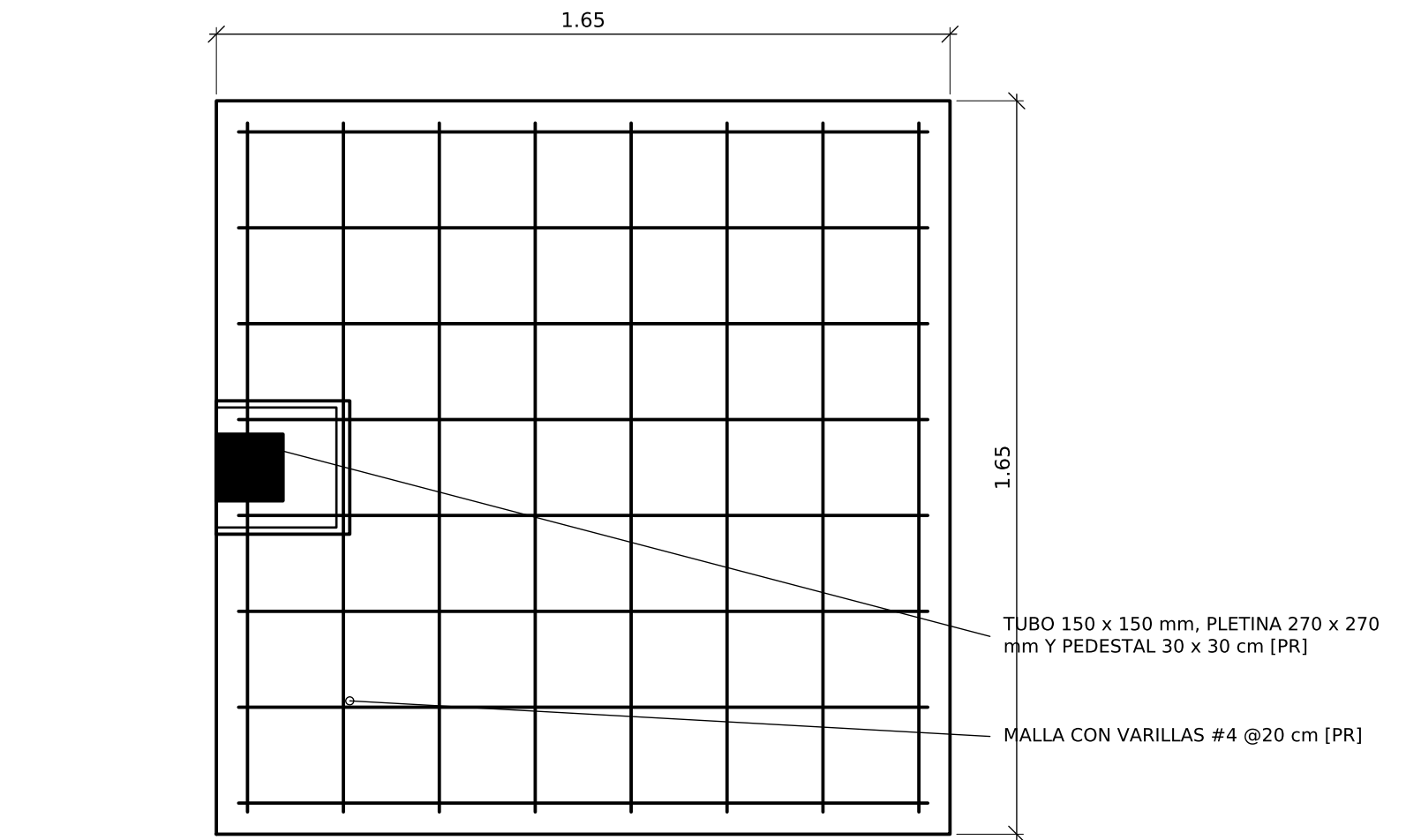
PLANTA FUNDACIÓN F2 Esc. 1:15
