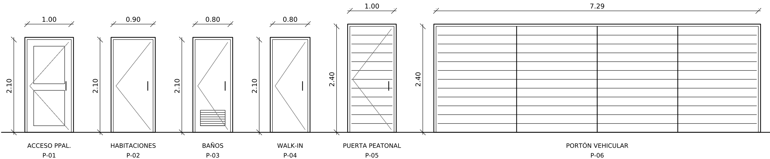
DETALLE PUERTAS
