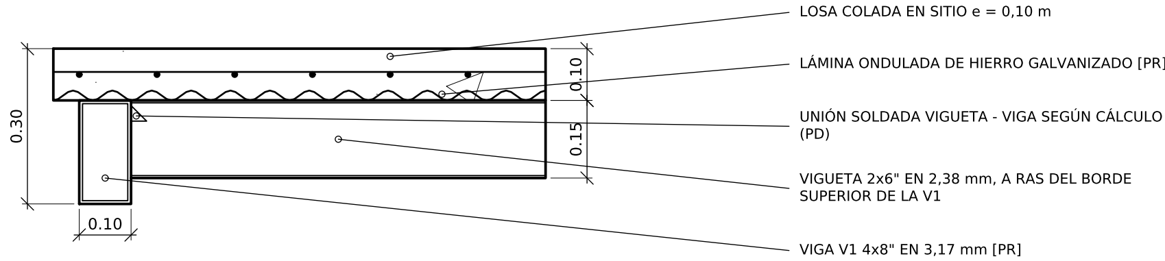
SECCIÓN A-A A LO LARGO DE LA VIGUETA - Esc. 1:10
