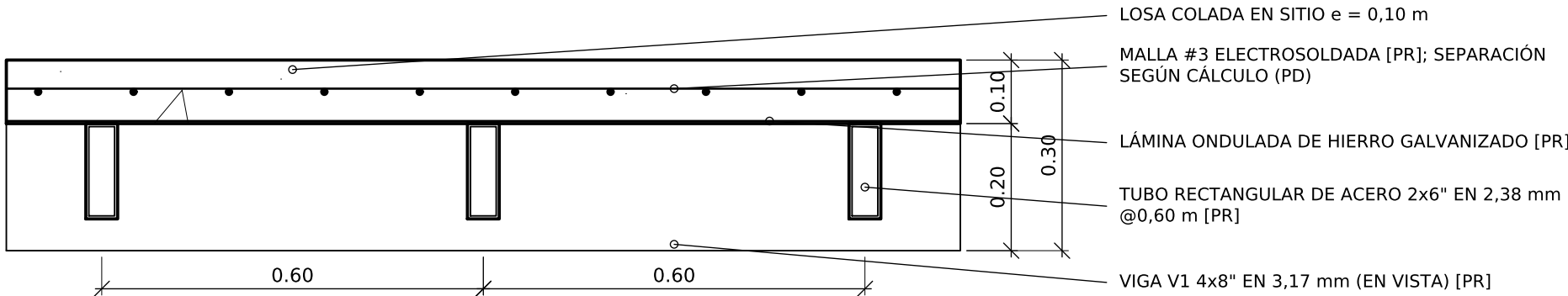
DETALLE DE ENTREPISO CORTE PERPENDICULAR A LAS VIGUETAS - Esc. 1:10
