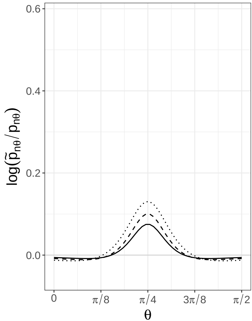
t_4 copula
