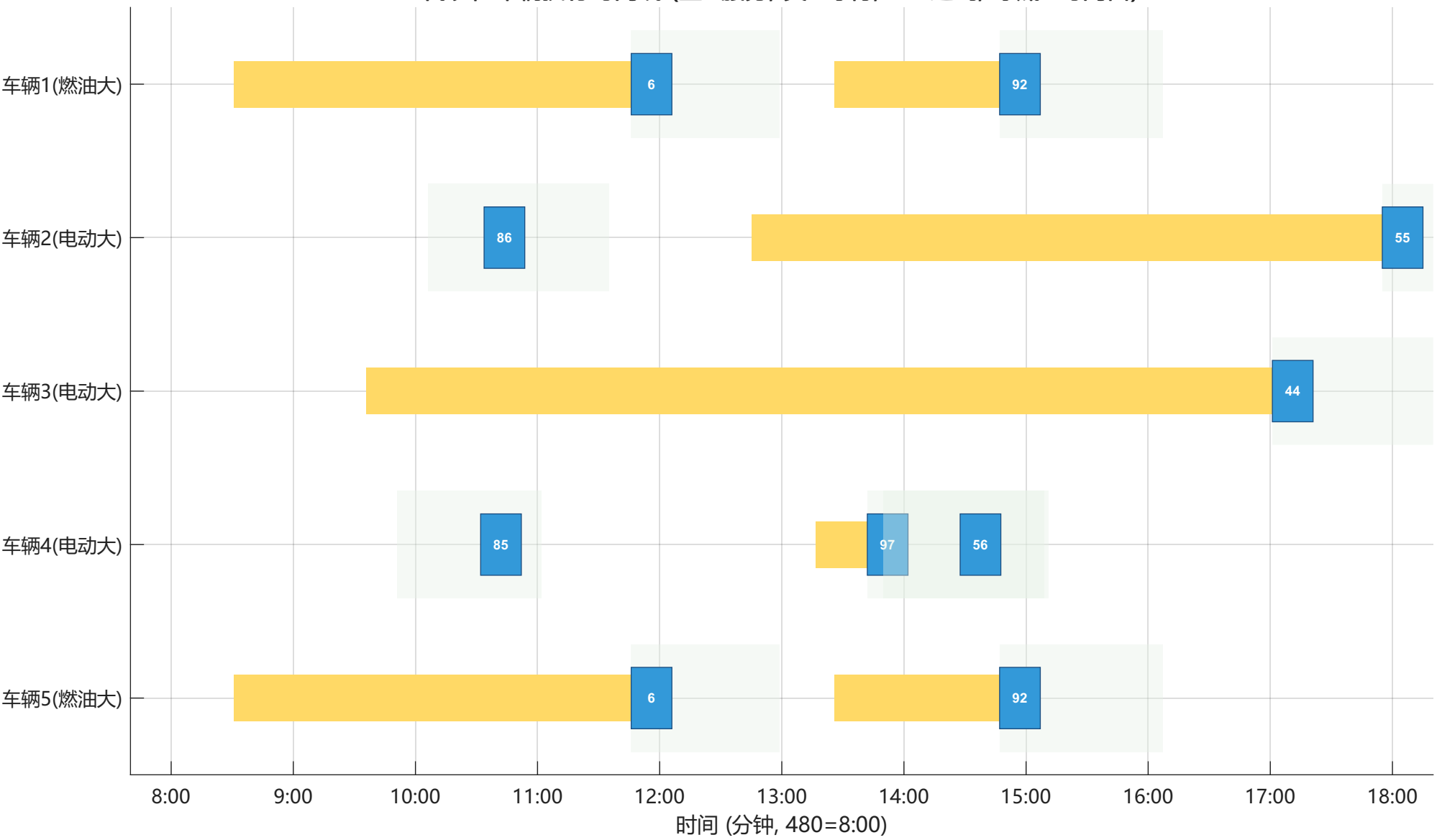
代表性车辆执行时间线 (蓝=服务, 黄=等待, 红=迟到, 绿底=时间窗)
