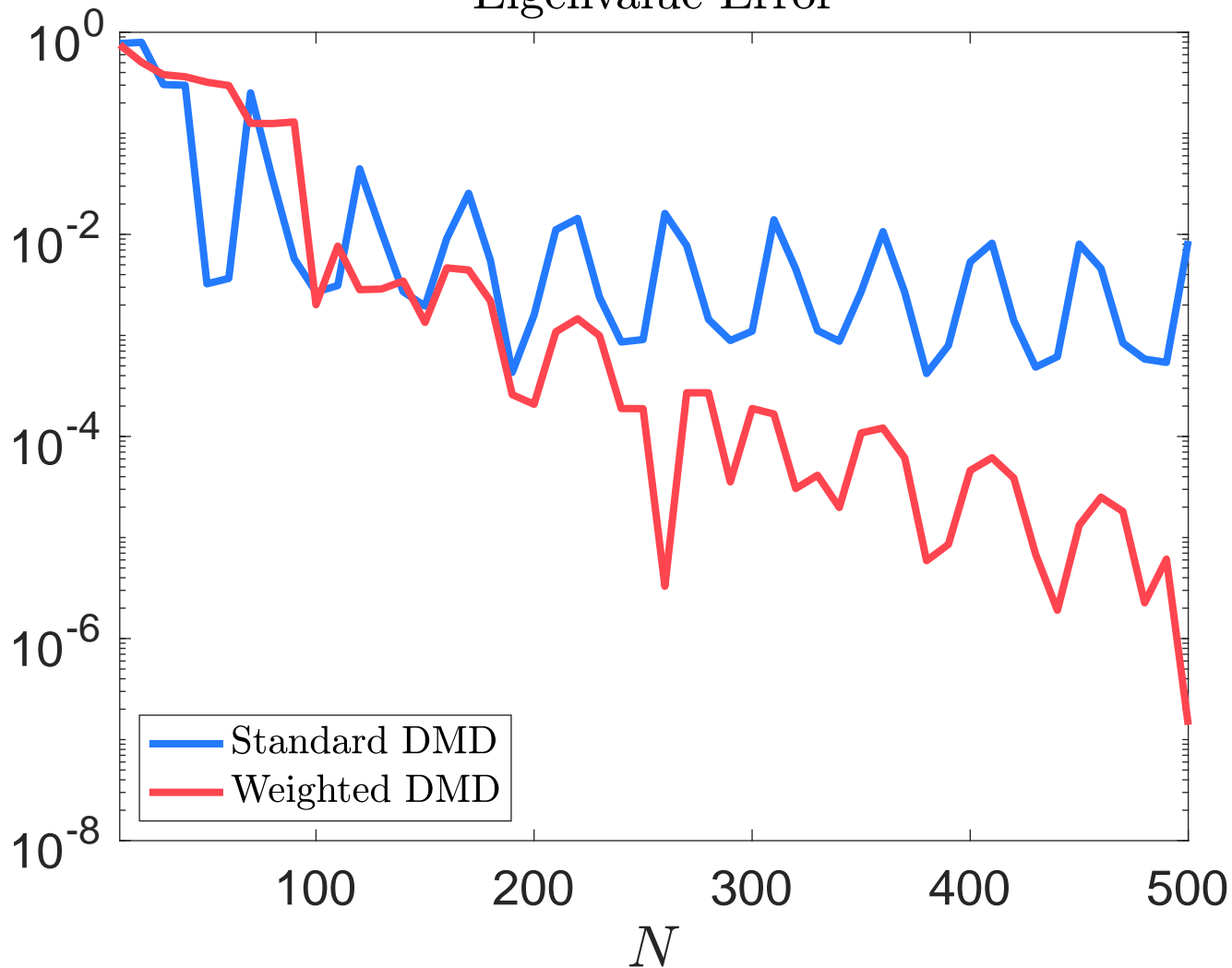
Eigenvalue Error
