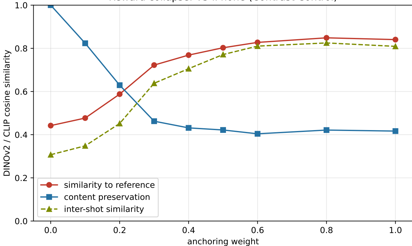
Reward collapse: V5 iPhone (Contrast Control)
