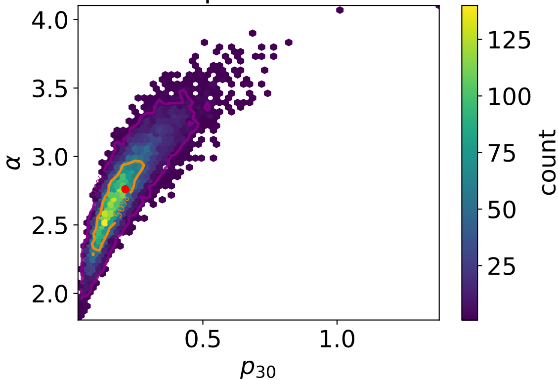
Population 4
