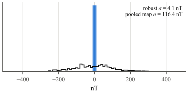
(d) RM3100 magnetic
