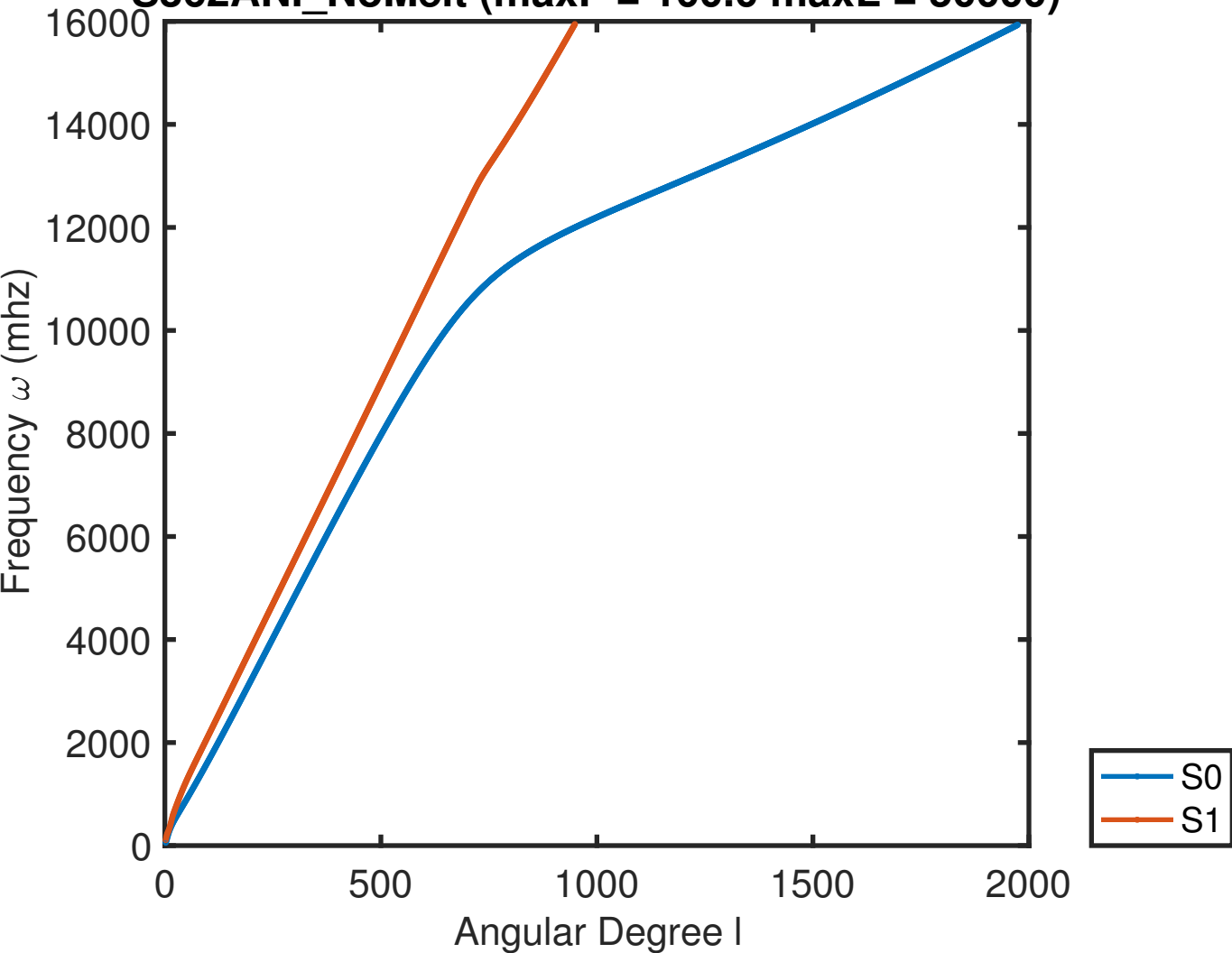
S362ANI_NoMelt (maxF = 100.0 maxL = 50000)
