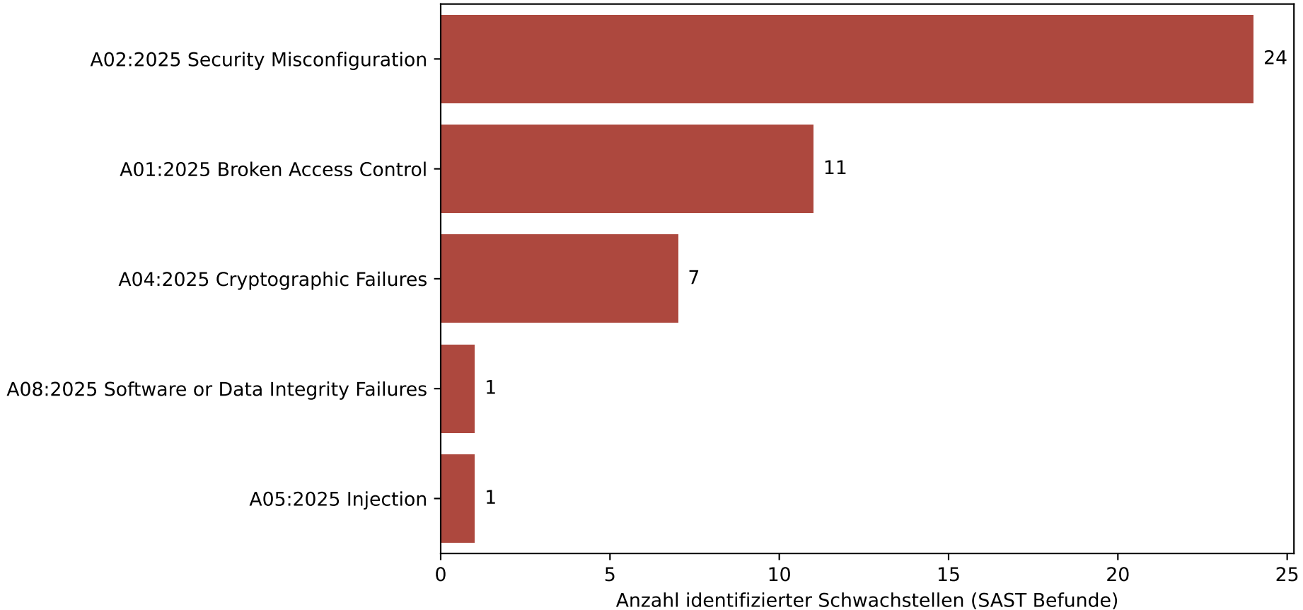
Prädominanz der OWASP-Kategorien über alle evaluierten Modelle
