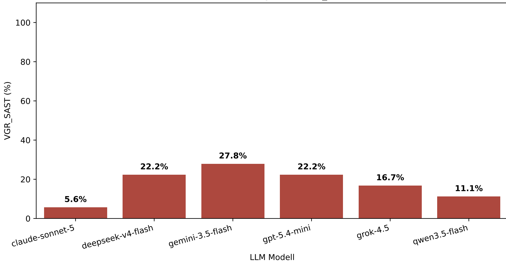
Gesamte Schwachstellen-Generierungsrate (VGR_SAST) im Baseline-Szenario
