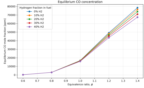
(b) Equilibrium CO.
