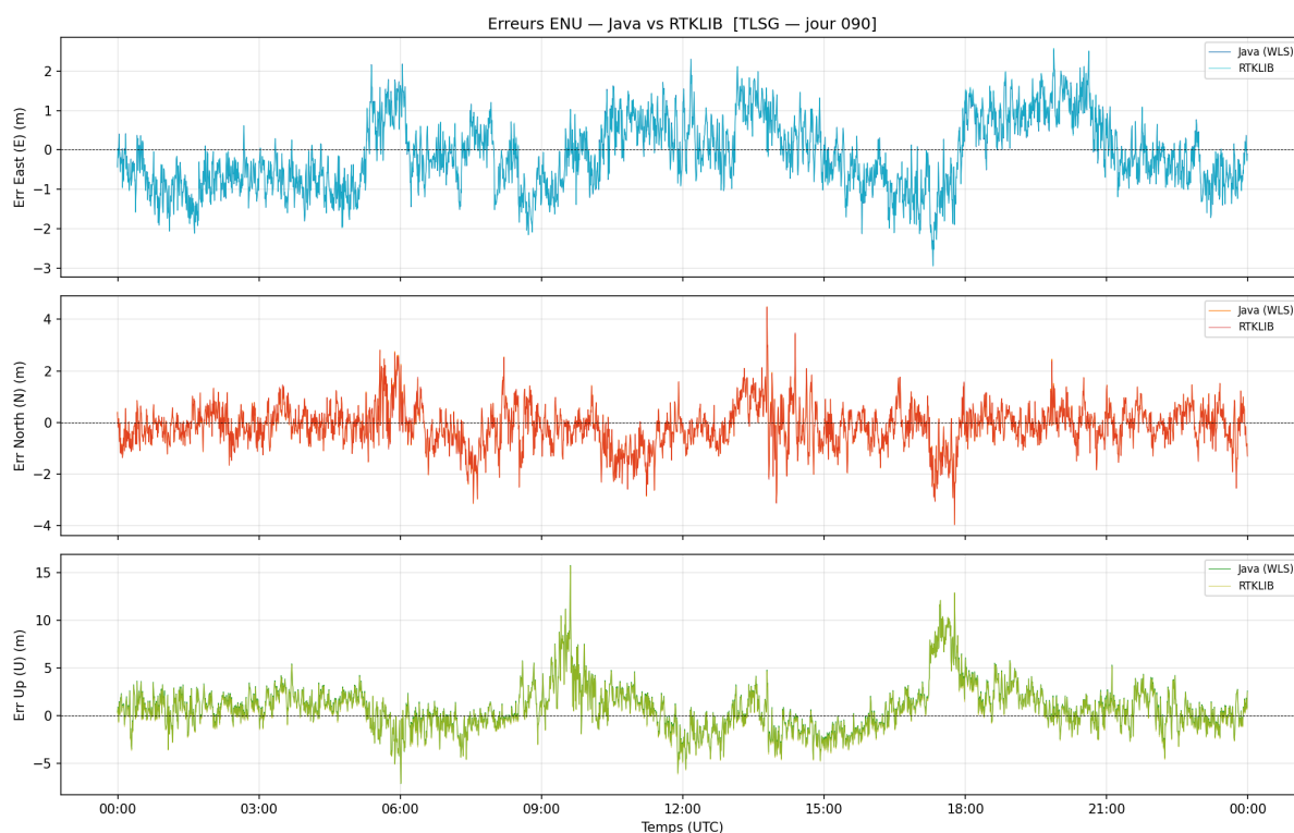
FIGURE 2.1 – Évolution des erreurs ENU de la configuration SPP témoin.
