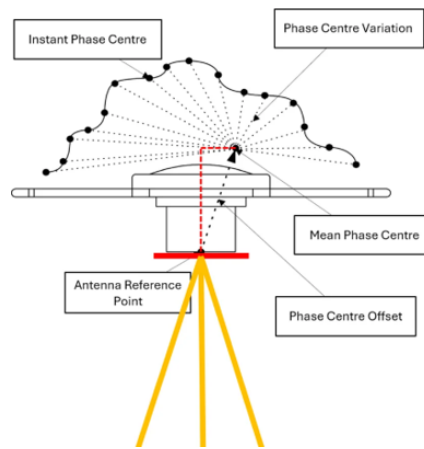
FIGURE 1.4 – Schéma illustrant le décalage PCO/PCV d'une antenne et son centre de phase.
