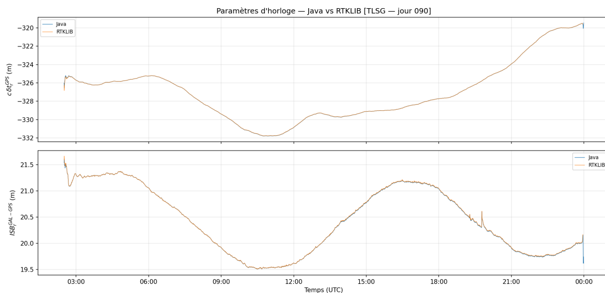
FIGURE 2.17 – Horloge GPS du récepteur et ISB GALILEO-GPS estimés par Java et RTKLIB.
