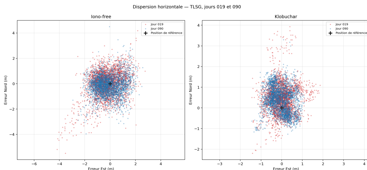
FIGURE 2.8 – Dispersion horizontale aux jours 019 et 090 avec les modèles IF et Klobuchar.
