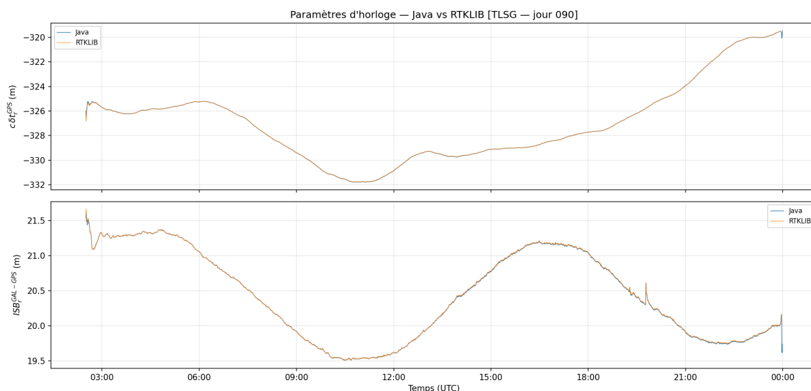
FIGURE 2.16 – Horloge GPS du récepteur et ISB GALILEO-GPS estimés par Java et RTKLIB.
