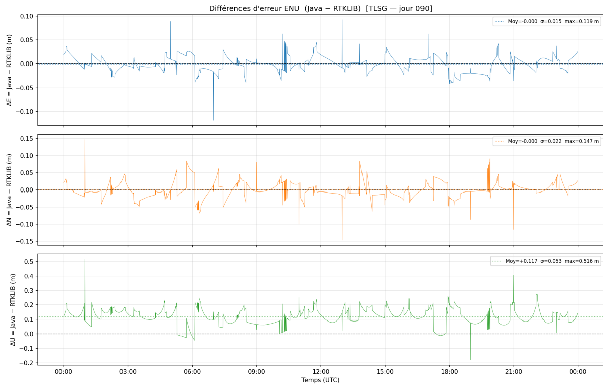
FIGURE 2.2 – Différences ENU entre Java-Orekit et RTKLIB pour la configuration SPP témoin.
