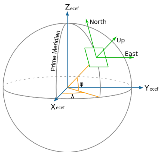
FIGURE 1.2 – Définition des axes du repère ECEF et ENU. Source : DIRSIG, Rochester Institute of Technology.
