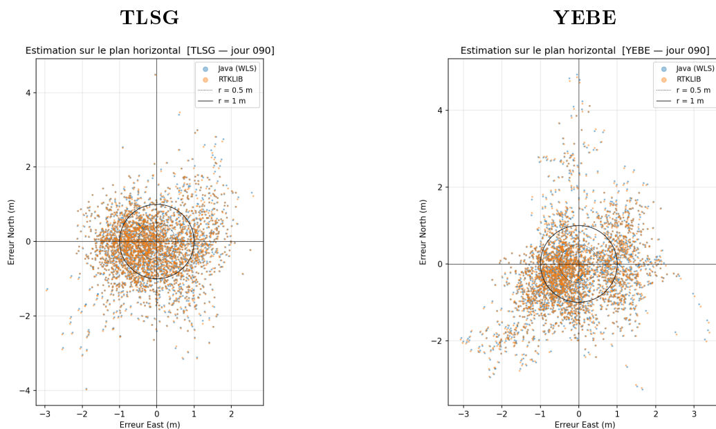
FIGURE 2.7 – Influence de la station sur la dispersion horizontale de la solution SPP.
