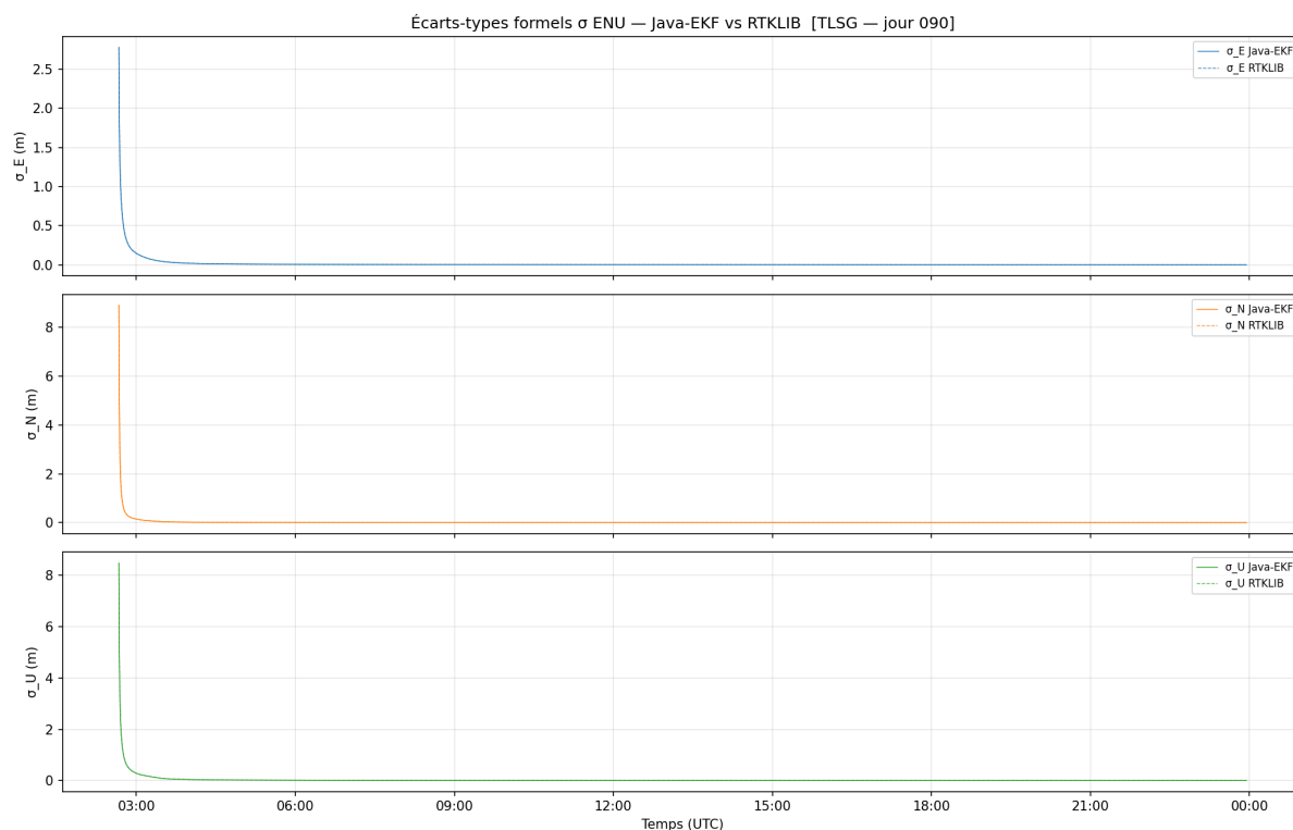
FIGURE 2.12 – Écart-types formels ENU du PPP précis.
