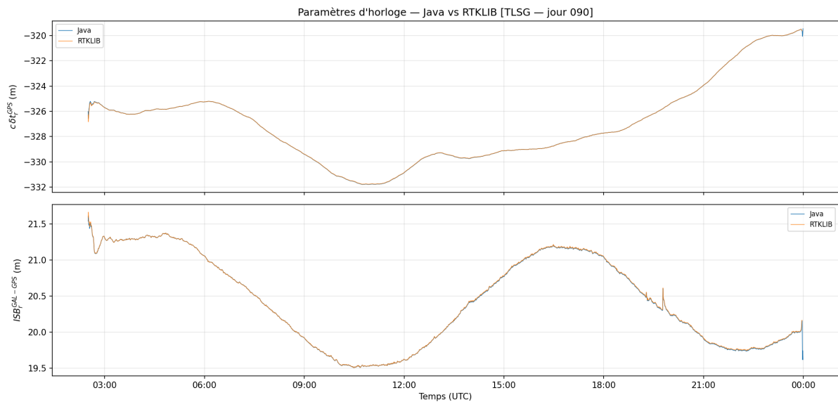
FIGURE 2.17 – Horloge GPS du récepteur et ISB GALILEO-GPS estimés par Java et RTKLIB.
