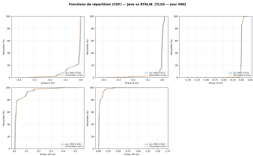
FIGURE 2.16 – Fonctions de répartition des erreurs du PPP précis GPS+GALILEO.
