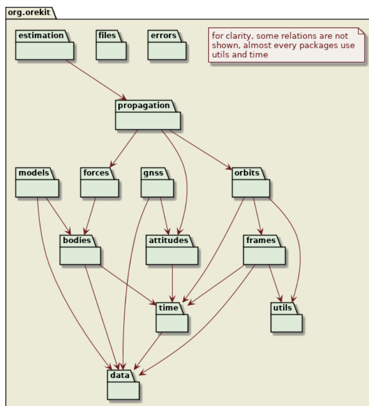
FIGURE 1.4 – Organisation des principaux packages d'Orekit. Source : Orekit, Overview.
