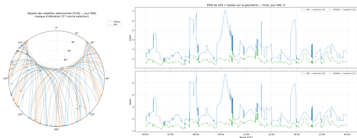
FIGURE 2.5 – Répartition des satellites et effet de l'ajout de GALILEO sur le GDOP et le PDOP à TLSG.
