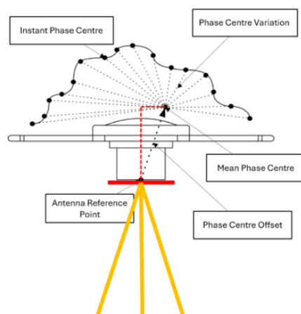
FIGURE 1.3 – Schéma illustrant le décalage PCO/PCV d'une antenne. Source : Maile et al. [?].
