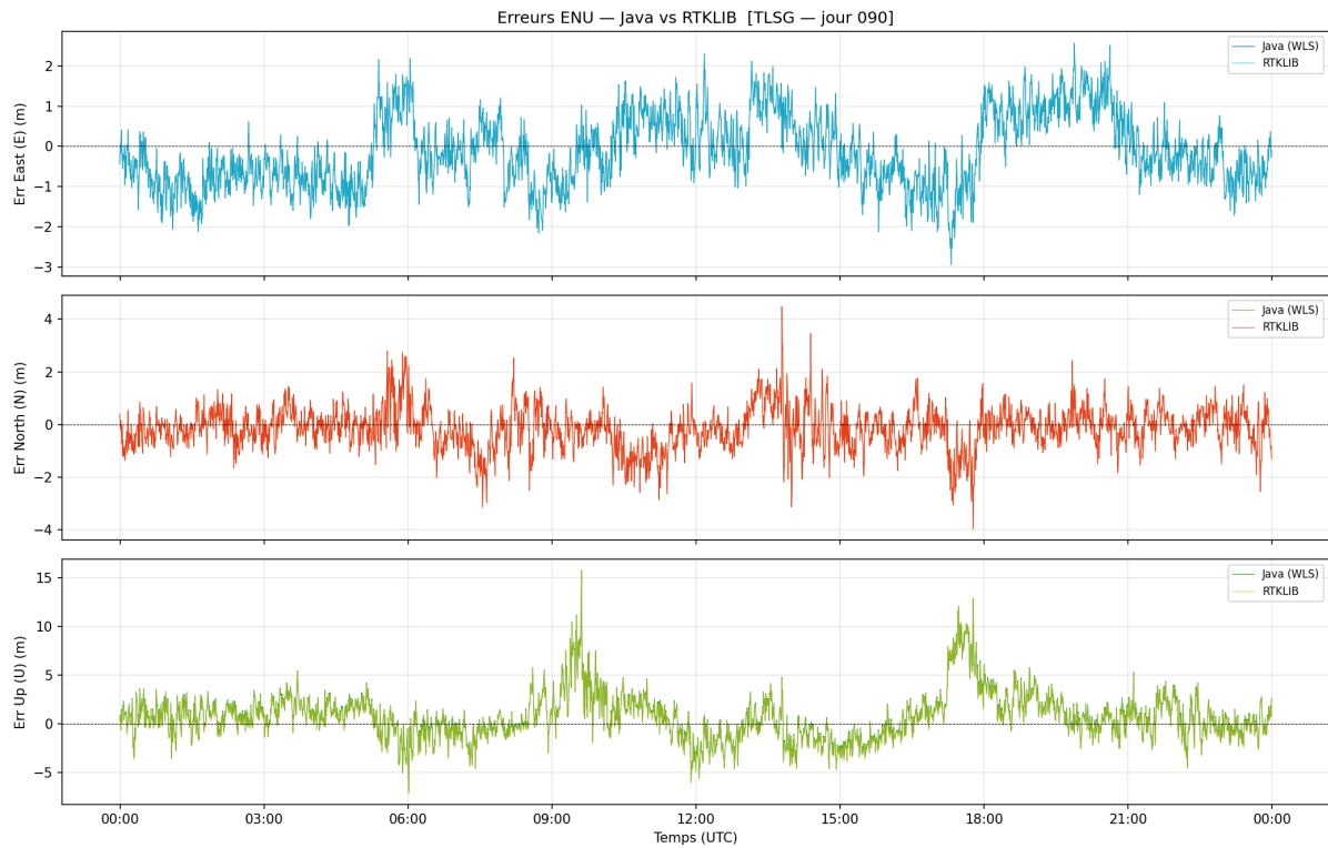
FIGURE 2.2 – Évolution des erreurs ENU de la configuration SPP témoin.
