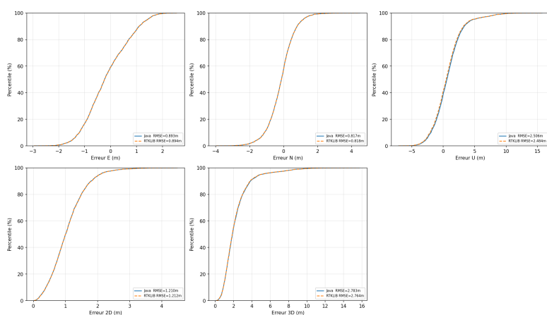
FIGURE 2.4 – Fonctions de répartition des erreurs avec les traitements ionosphériques IF et Klobuchar.
