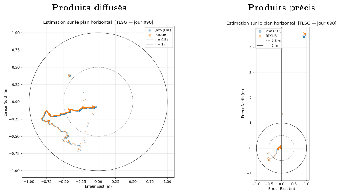
FIGURE 2.14 – Dispersion horizontale de l'EKF avec les produits diffusés et précis.
