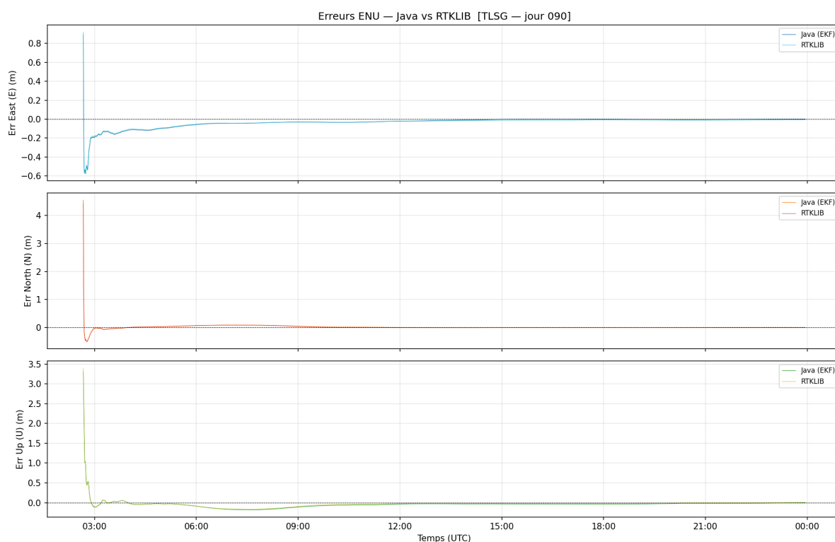
FIGURE 2.10 – Convergence des erreurs ENU du PPP précis à TLSG.
