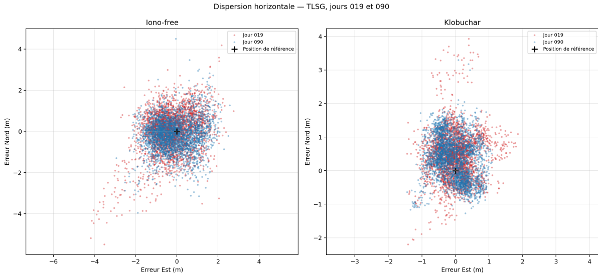
FIGURE 2.8 – Dispersion horizontale aux jours 019 et 090 avec les modèles IF et Klobuchar.
