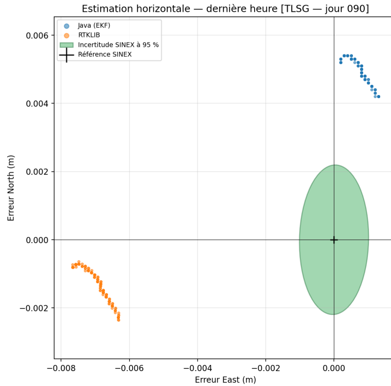
FIGURE 2.11 – Dispersion horizontale pendant la dernière heure du PPP précis GPS.
