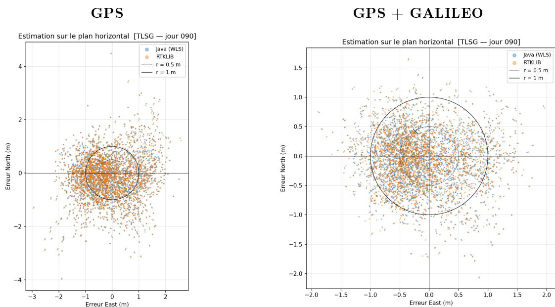
FIGURE 2.6 – Effet de l'ajout de GALILEO sur la solution SPP à TLSG.
