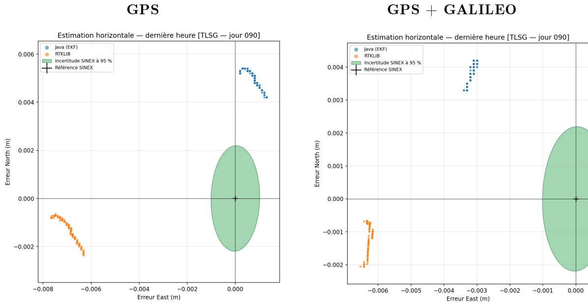
FIGURE 2.15 – Effet de GALILEO sur la dispersion horizontale du PPP précis pendant la dernière heure.
