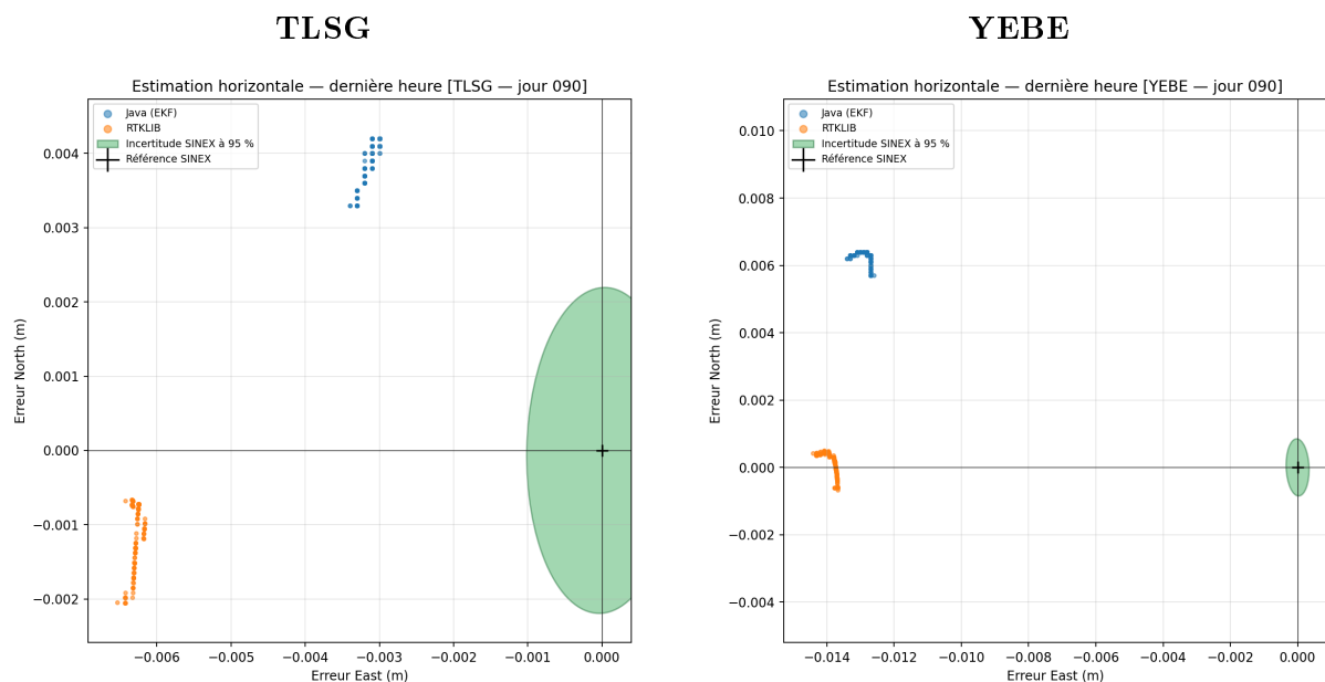
FIGURE 2.18 – Dispersion horizontale du PPP précis GPS+GALILEO à TLSG et YEBE pendant la dernière heure.
