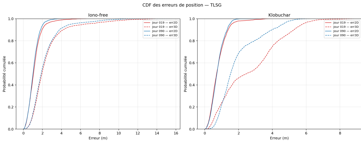
FIGURE 2.9 – Fonctions de répartition des erreurs aux jours 019 et 090.
