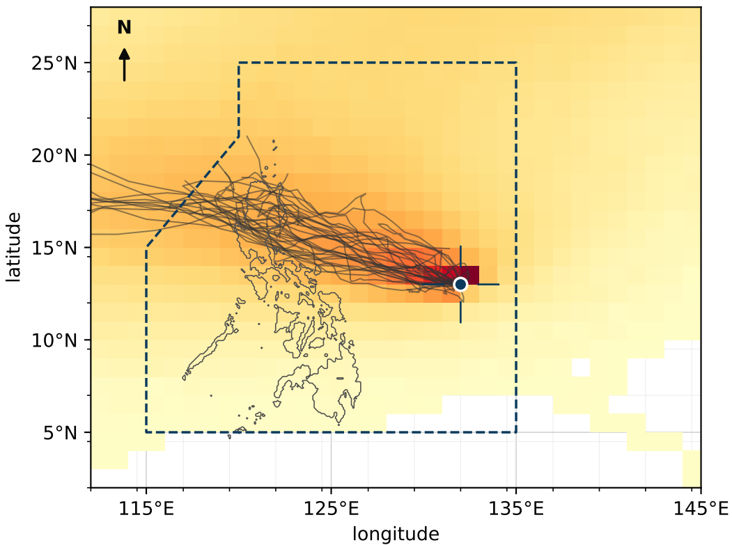
(a) 13°N, 132°E, October, inside PAR
