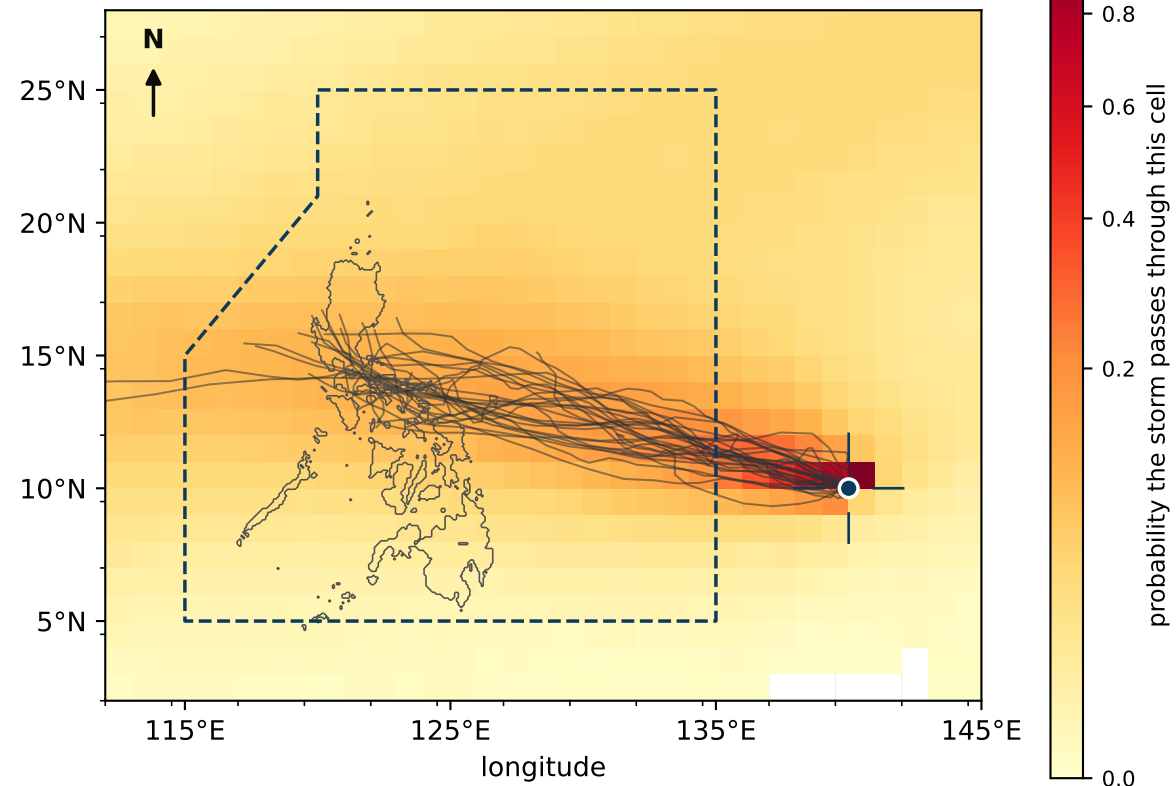
(b) 10°N, 140°E, November, outside PAR
