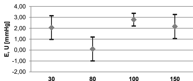
ERROR E INCERTIDUMBRE EXPANDIDA PRESIÓN DIASTÓLICA NO INVASIVA
