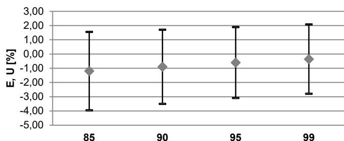
ERROR E INCERTIDUMBRE EXPANDIDA SATURACIÓN PARCIAL DE OXÍGENO
