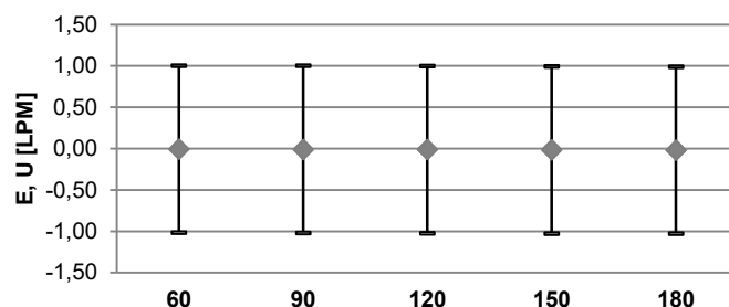
ERROR E INCERTIDUMBRE EXPANDIDA FRECUENCIA CARDÍACA
