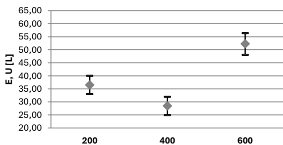
ERROR E INCERTIDUMBRE EXPANDIDA Vt
