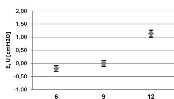
ERROR E INCERTIDUMBRE EXPANDIDA PEEP
